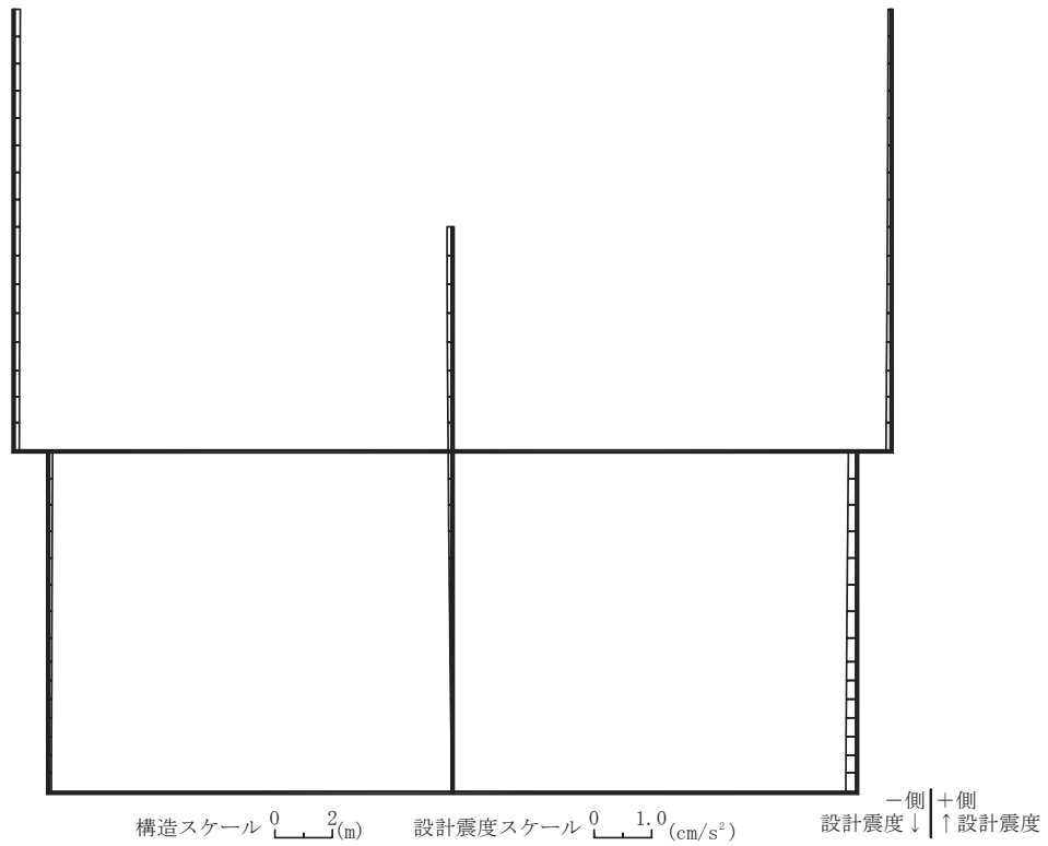
図 3-14 作用荷重分布図 (設計震度分布) (解析ケース③, S s - N 1 (++) , C-C 断面, 東西 (循環水ポンプエリア))
