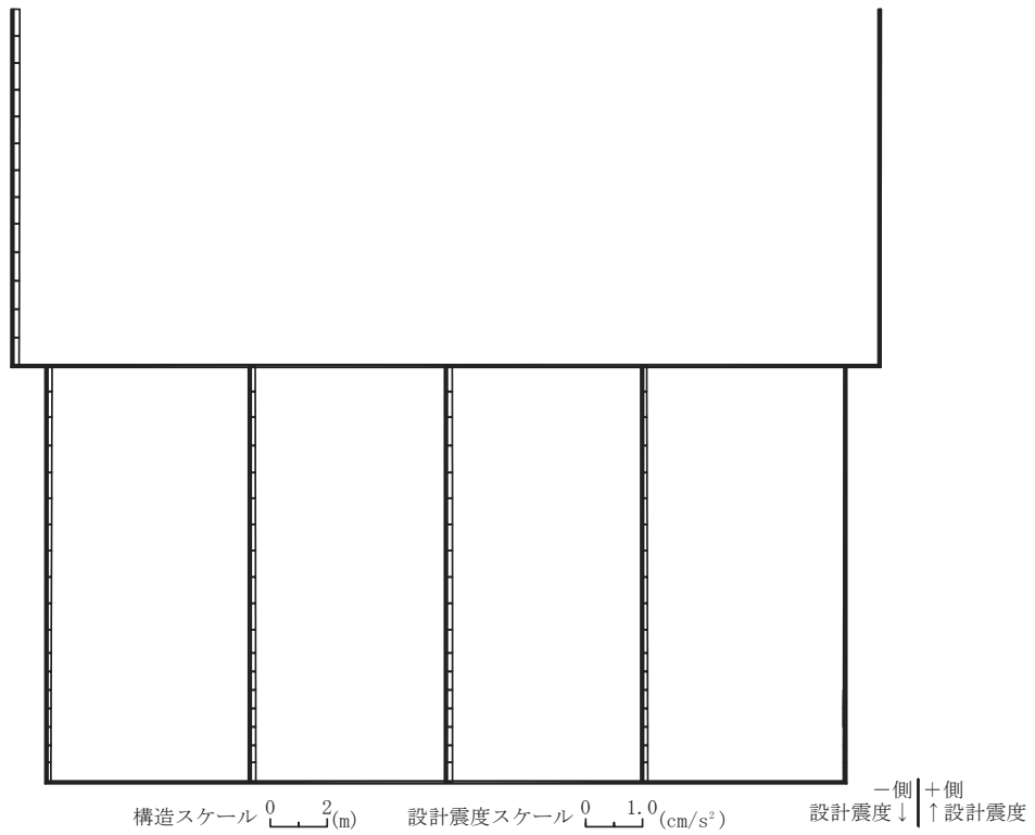
図 3-12 作用荷重分布図 (設計震度分布)
