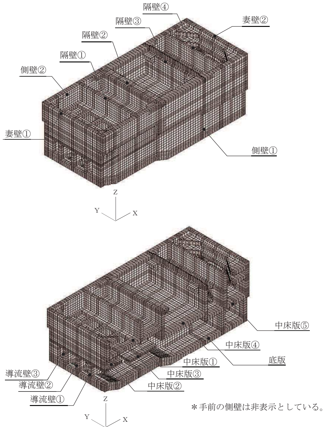
図4-1 各部材位置
