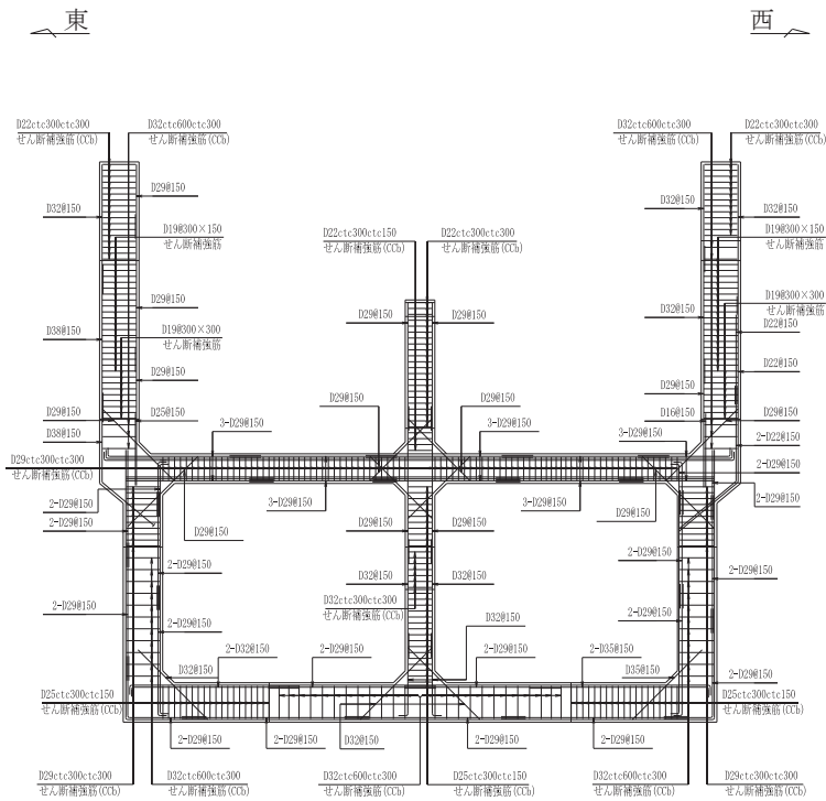
図 2-9 海水ポンプ室概略配筋図 (C-C 断面)
