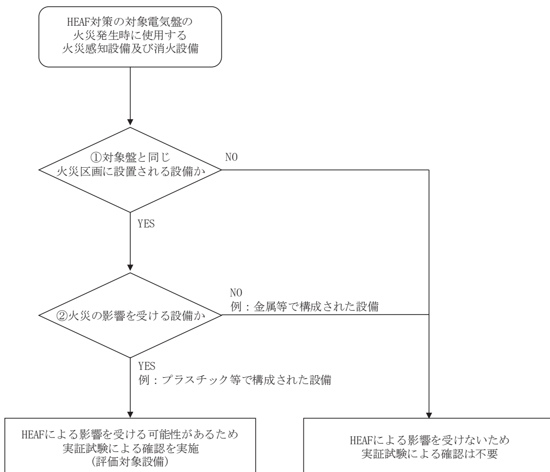
図 6.8 評価対象設備の選定フロー
