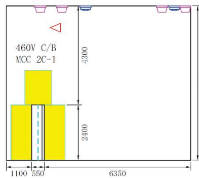
A-A' 断面
