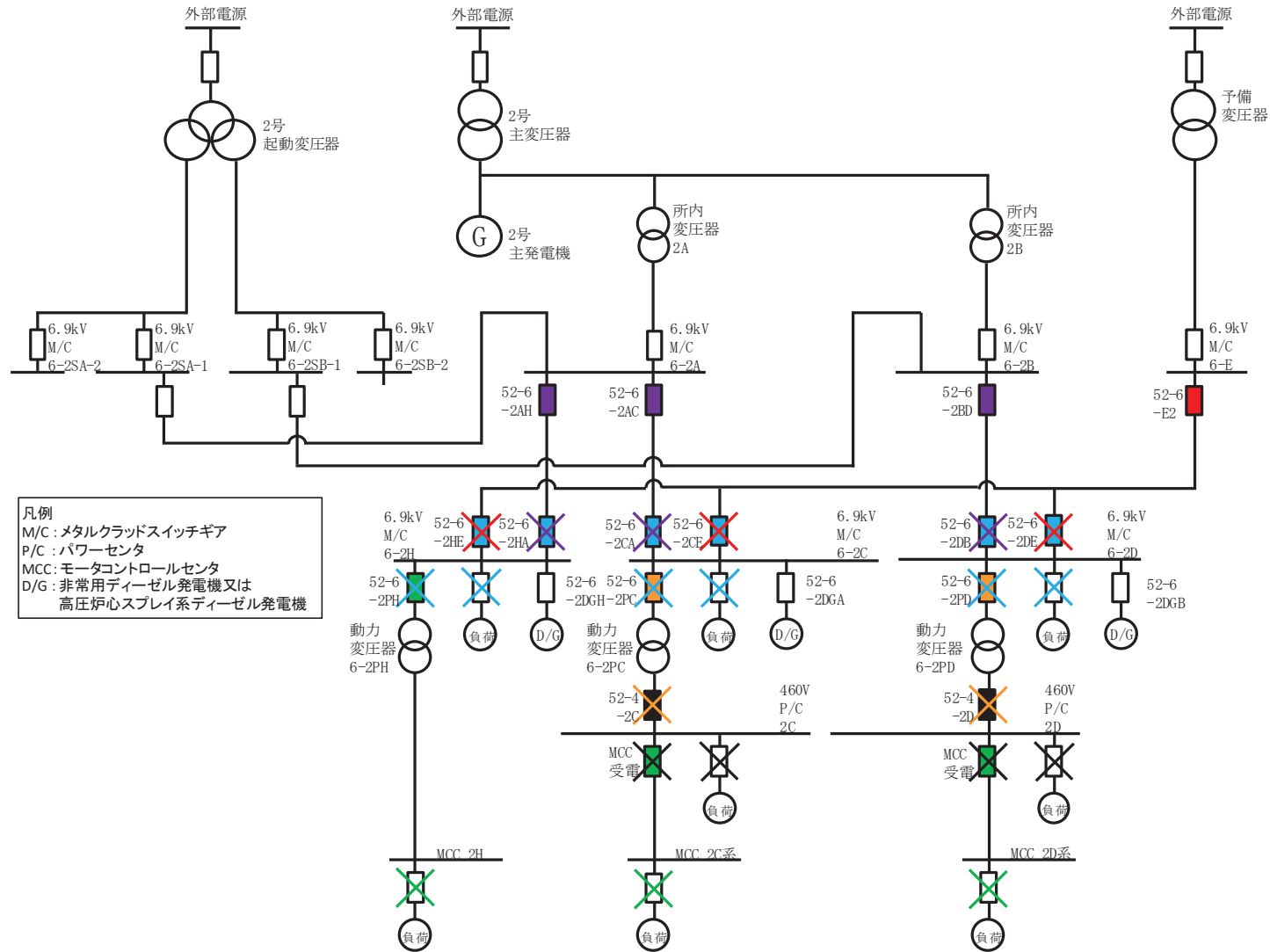
図 3.2 HEAF 対策が必要な電気盤系統図 (1/2)
