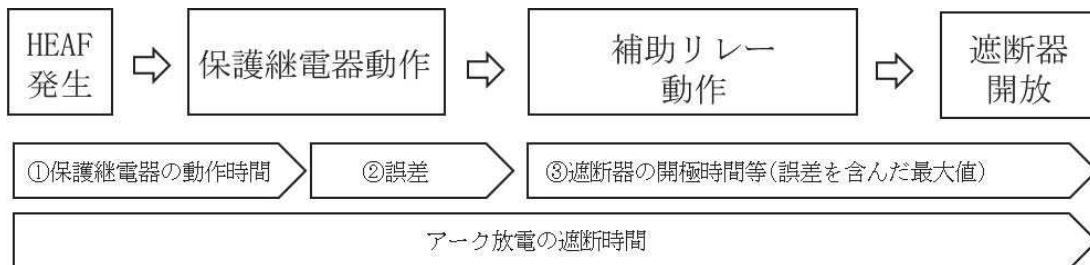
図 6.2 アーク放電の遮断時間に含まれる誤差の考え方(1/2)
