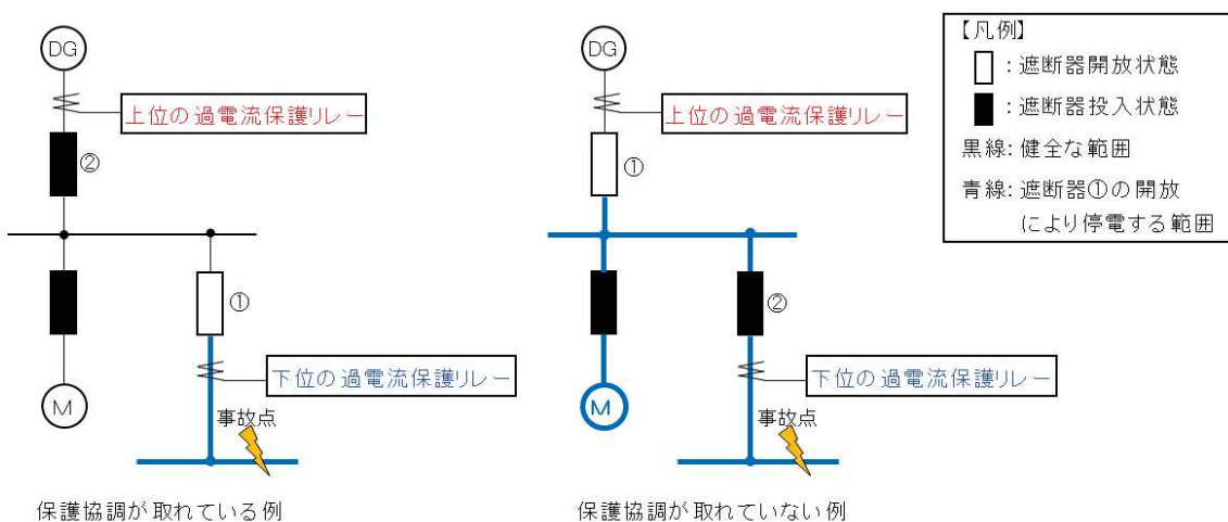
図 6.3 保護協調のイメージ
