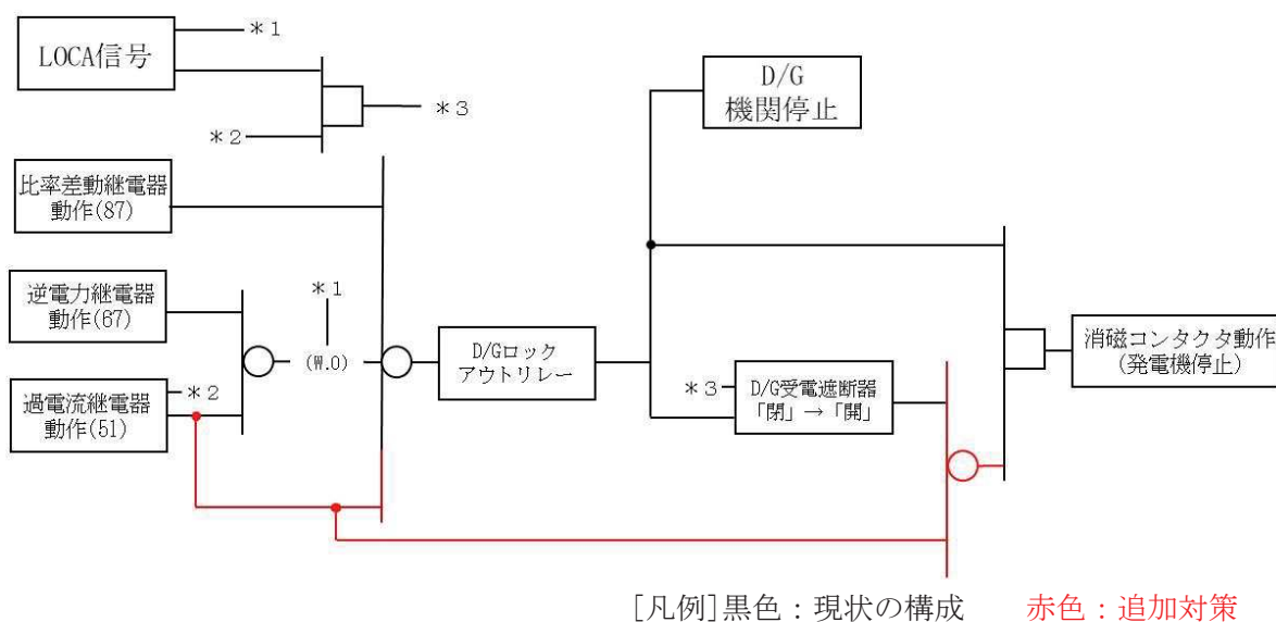
図 5-3 51要素をD/G停止インターロックに追加した場合のインターロックイメージ
