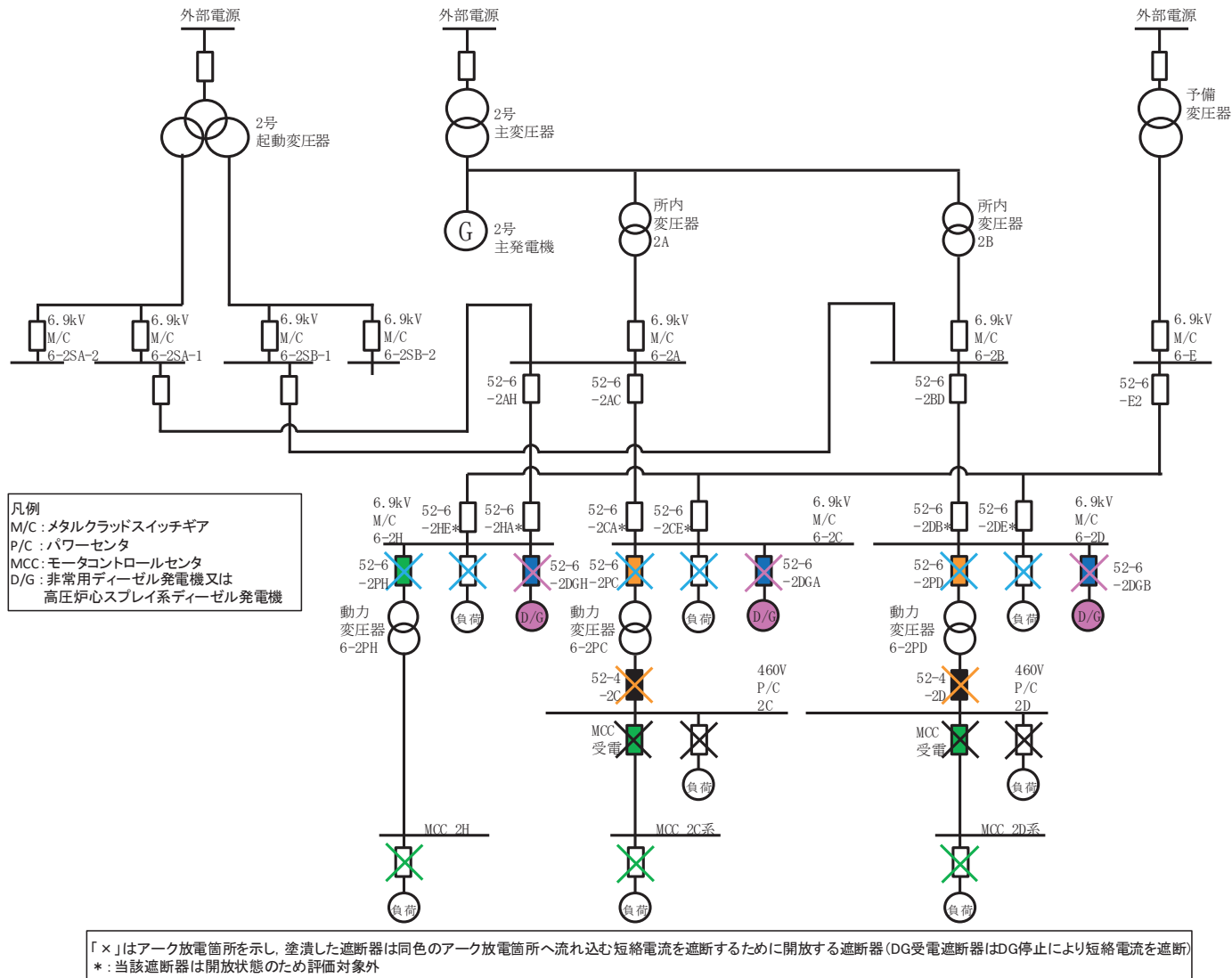
図 3.2 HEAF 対策が必要な電気盤系統図 (2/2) (非常用ディーゼル発電機又は高圧炉心スプレイ系ディーゼル発電機からの給電時)
