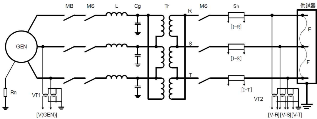
図 4. 3. 2 P/C 試験回路
