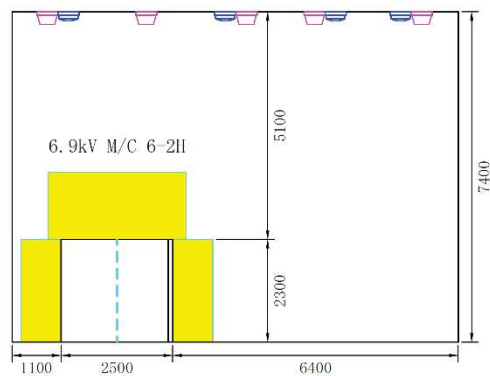
A-A' 断面
