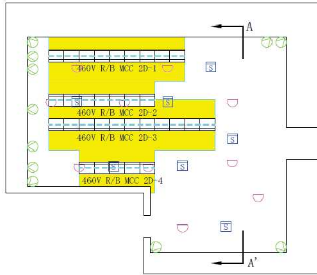
区分Ⅱ非常用MCC室 平面図 (O.P. 6000)
