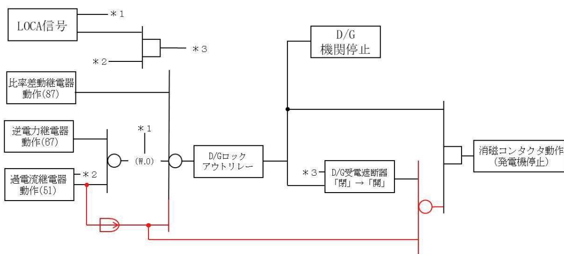
図 6.7 インターロック図 (概要)
