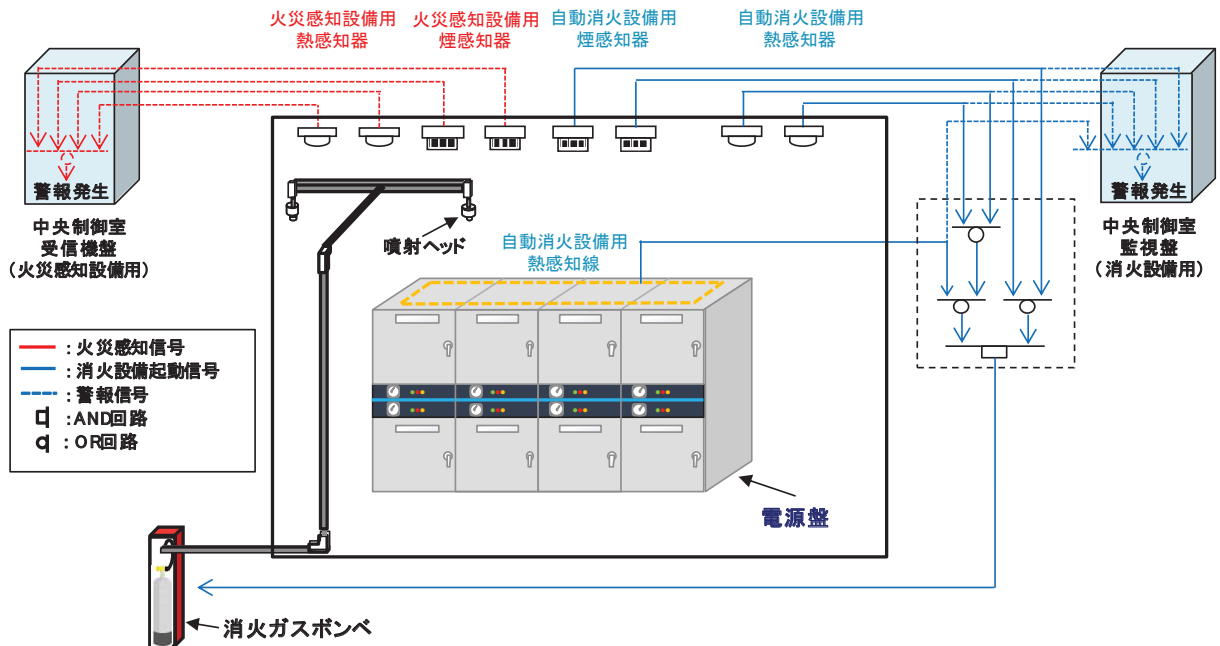
図 6.9 火災感知設備及び消火設備のシステム構成概要図
