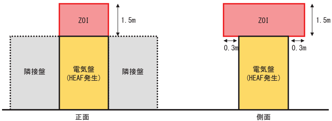
図 6.10 火災感知器に対する HEAF の ZOI
