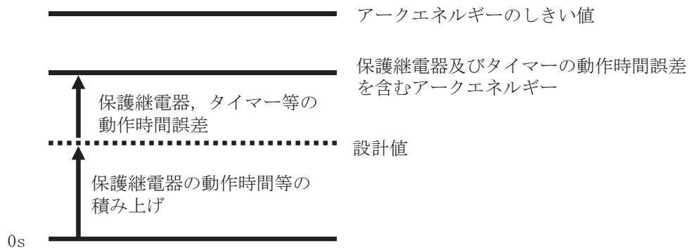
図 6.1 アーク放電の遮断時間の考え方
