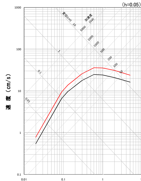
速度 (cm/s) 周期 (s) 応答スペクトル図(鉛直方向)
