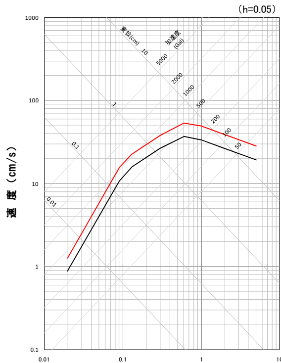
速度 (cm/s) 周期 (s) 応答スペクトル図(水平方向)
