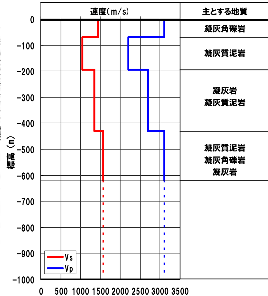
1号機原子炉建屋PS検層結果
