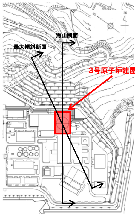
3号炉地盤モデル(断面位置)
