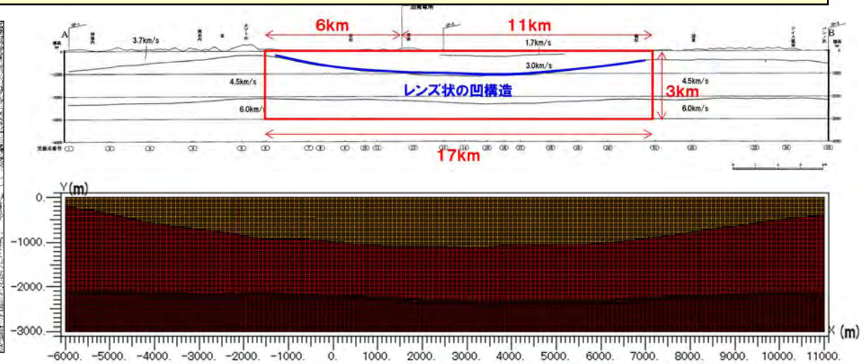
泊発電所 2次元FEMモデル
