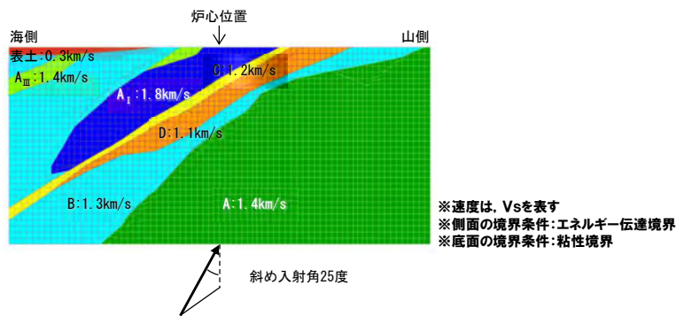
地盤モデル(最大傾斜断面)
