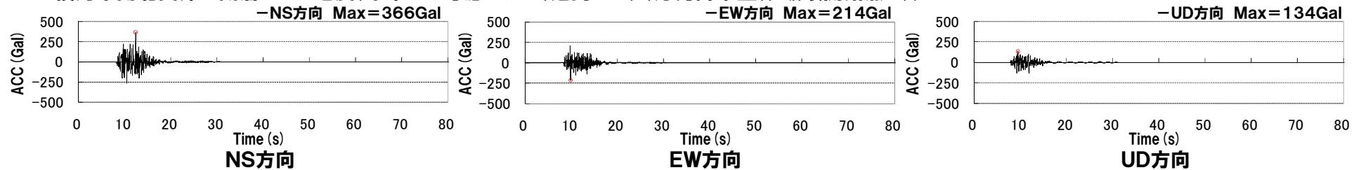
積丹半島北西沖の断層による地震(不確かさ考慮モデル(走向 0^{\circ} ))(応力降下量), 破壊開始点3))
