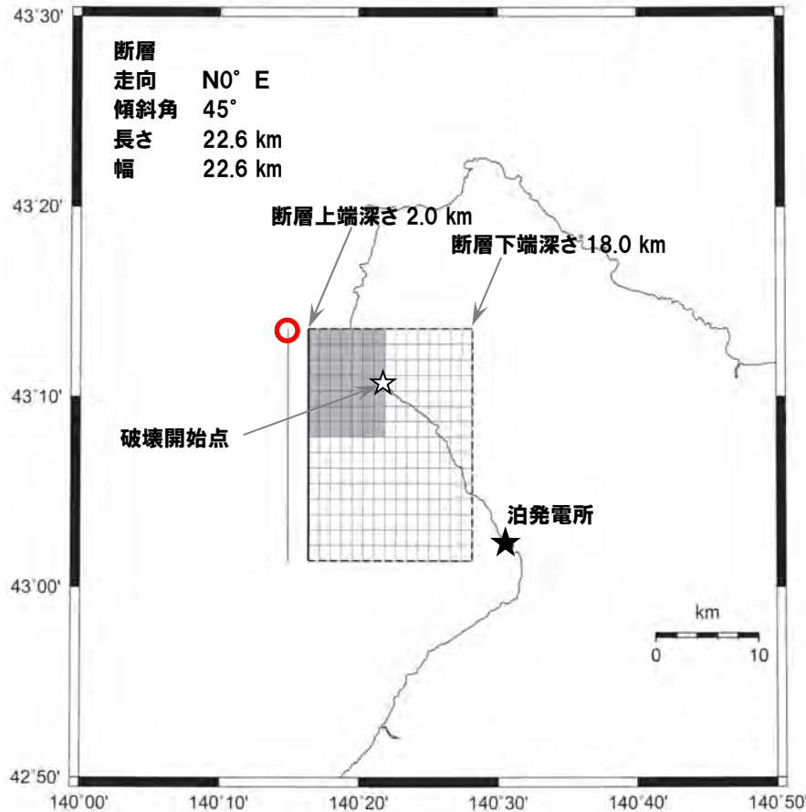
(積丹半島北西沖の断層による地震)震源モデル図, 断層パラメータ(基本震源モデル(走向0°))
