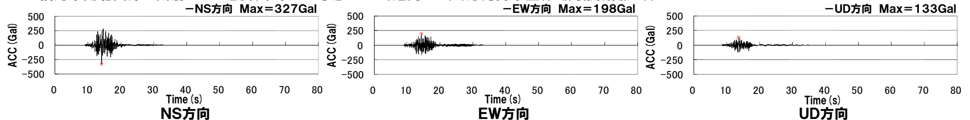
積丹半島北西沖の断層による地震(不確かさ考慮モデル(走向 0^{\circ} ))(応力降下量), 破壊開始点4))
