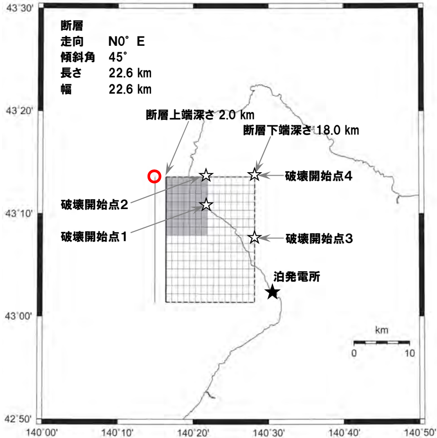
(積丹半島北西沖の断層による地震) 震源モデル図, 断層パラメータ(不確かさ考慮モデル(走向0°))(応力降下量)
