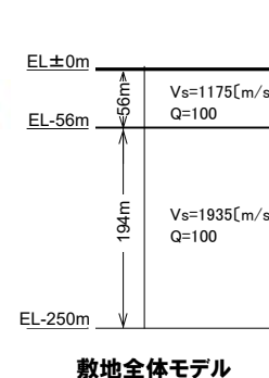
敷地全体モデル
