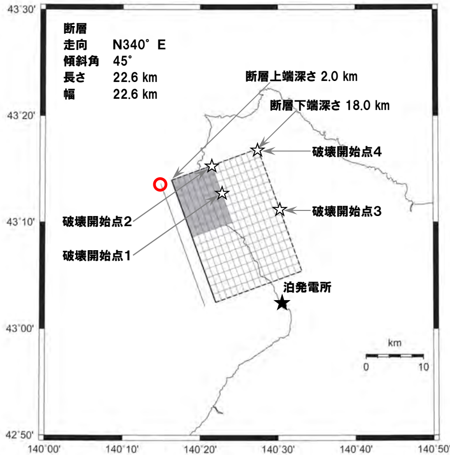
(積丹半島北西沖の断層による地震) 震源モデル図, 断層パラメータ(不確かさ考慮モデル(走向20°))(応力降下量)
