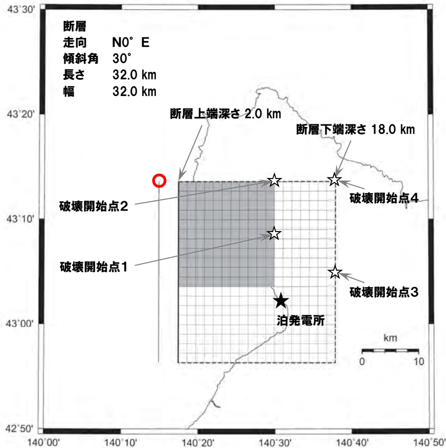
(積丹半島北西沖の断層による地震) 震源モデル図, 断層パラメータ(不確かさ考慮モデル(走向0°))(断層の傾斜角))
