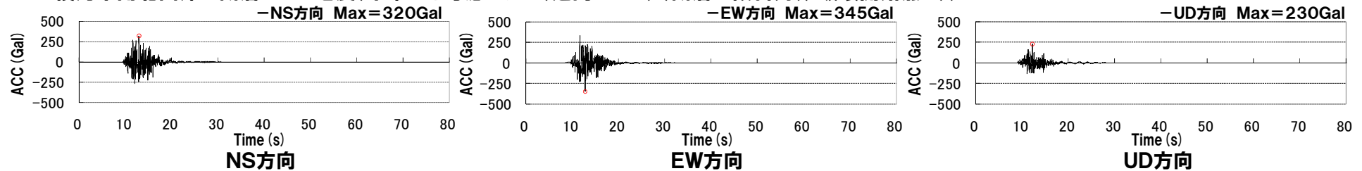
積丹半島北西沖の断層による地震(不確かさ考慮モデル(走向 20^\circ ))(断層の傾斜角), 破壊開始点3))
