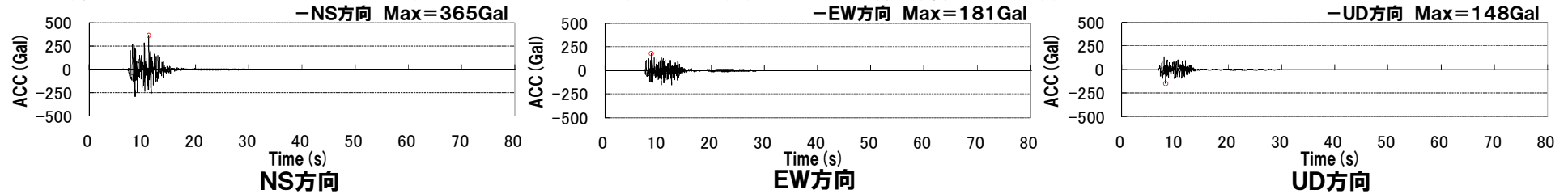
積丹半島北西沖の断層による地震(不確かさ考慮モデル(走向 0^{\circ} ))(応力降下量), 破壊開始点2))
