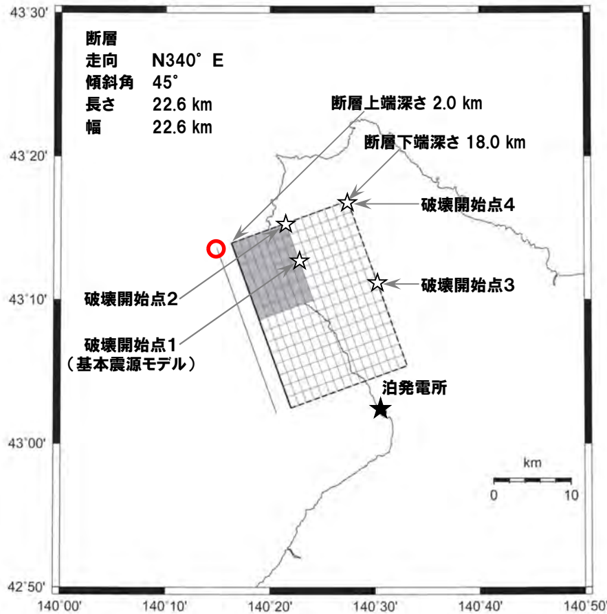
(積丹半島北西沖の断層による地震) 震源モデル図, 断層パラメータ(不確かさ考慮モデル(走向20°))(破壊開始点))
