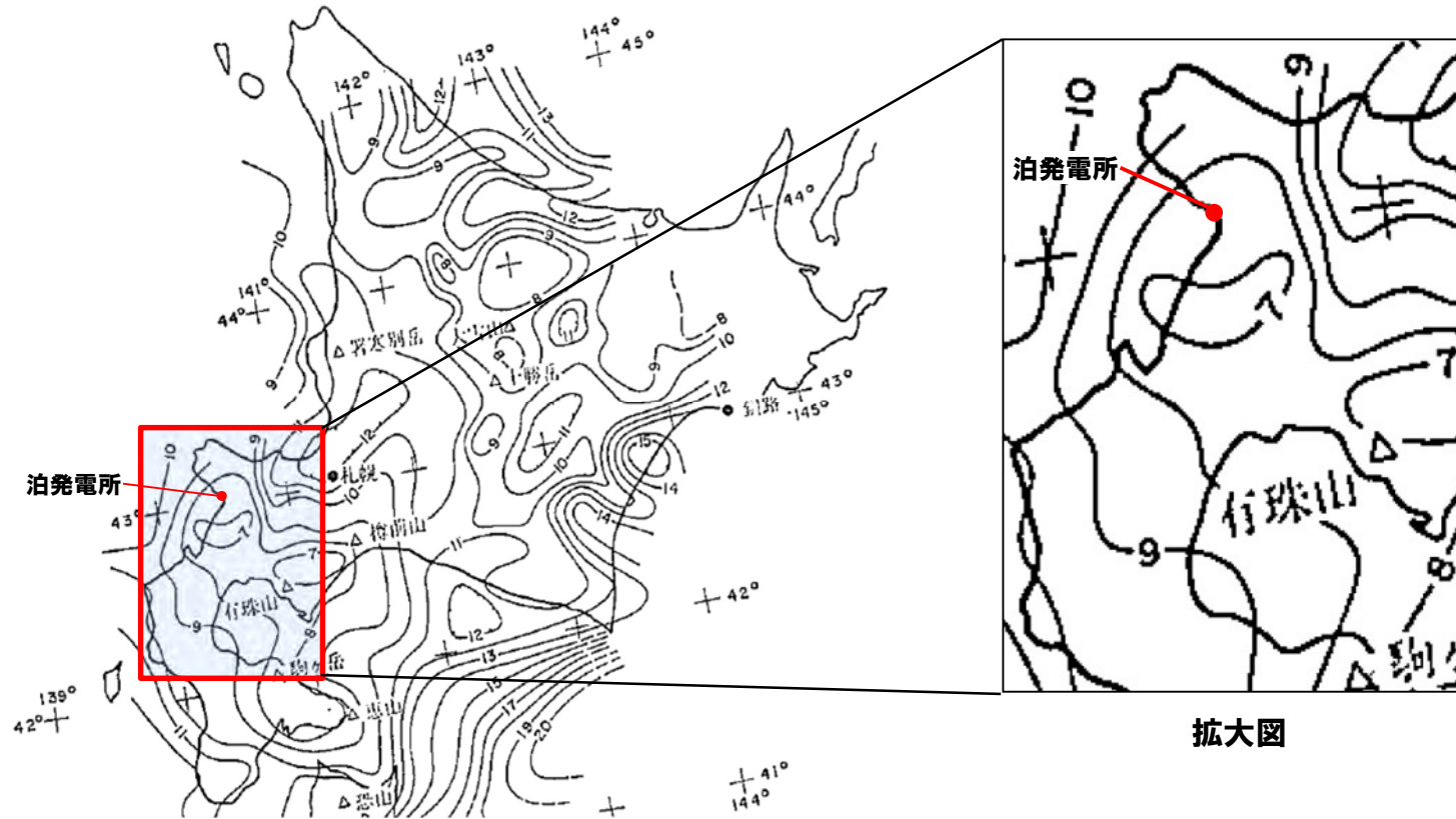
キュリー点深度分布(大久保(1984)に一部加筆)
