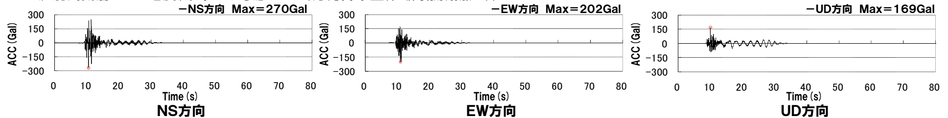
尻別川断層による地震(不確かさ考慮モデル(応力降下量), 破壊開始点3))
