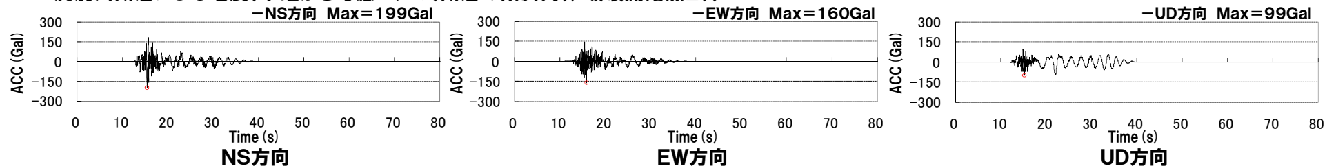
尻別川断層による地震(不確かさ考慮モデル(断層の傾斜角), 破壊開始点3))
