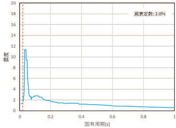
(鉛直方向)
