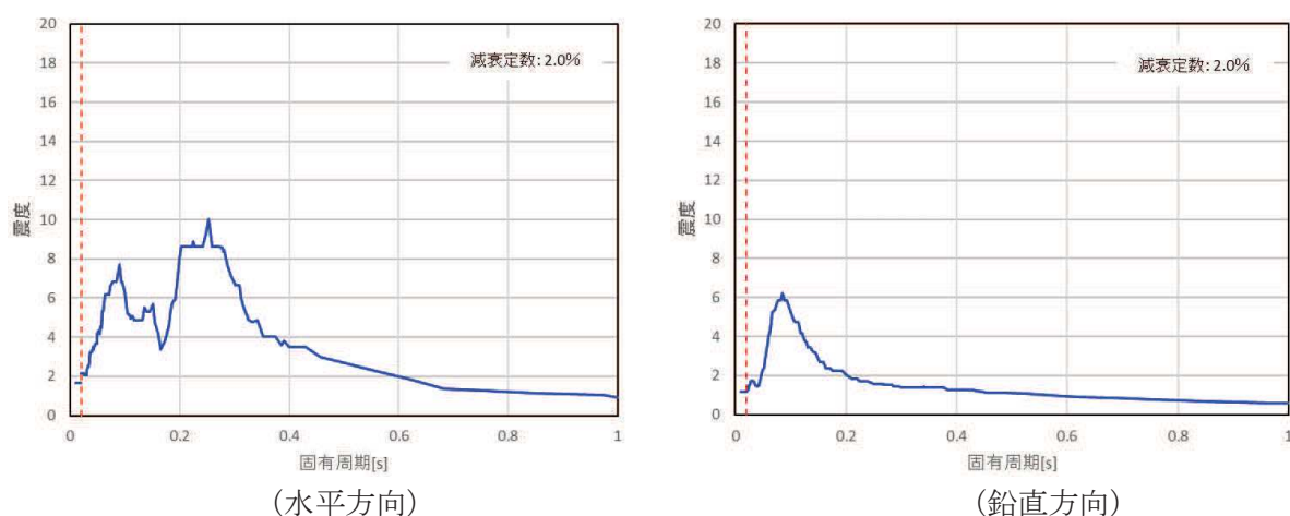
図 2-1 原子炉建屋 1F (O.P. 15.0m) の設計用床応答曲線 (減衰 2.0%, 固有周期 1.0 秒まで)
