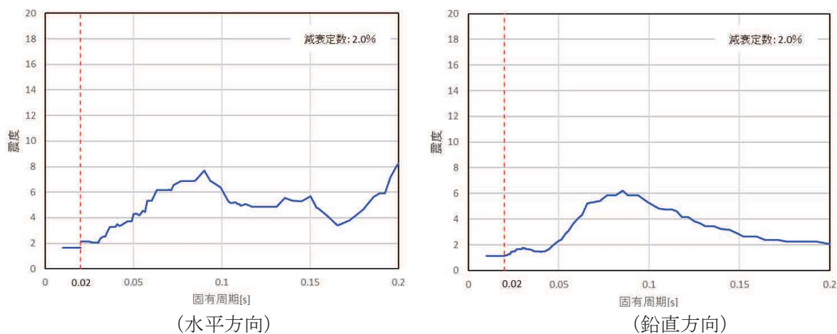
図 2-2 原子炉建屋 1F (O.P. 15.0m) の設計用床応答曲線 (減衰 2.0%, 固有周期 0.2 秒まで)
