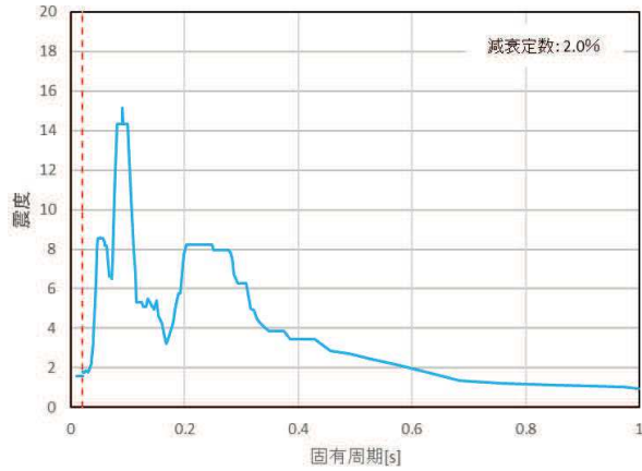
(水平方向)
