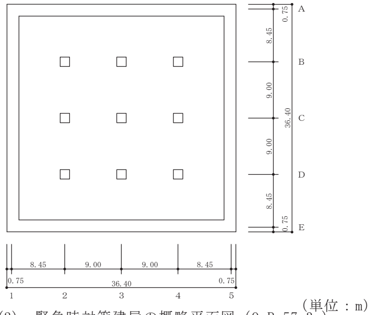
図 2-2(2) 緊急時対策建屋の概略平面図 (0.P. 57.3m)
