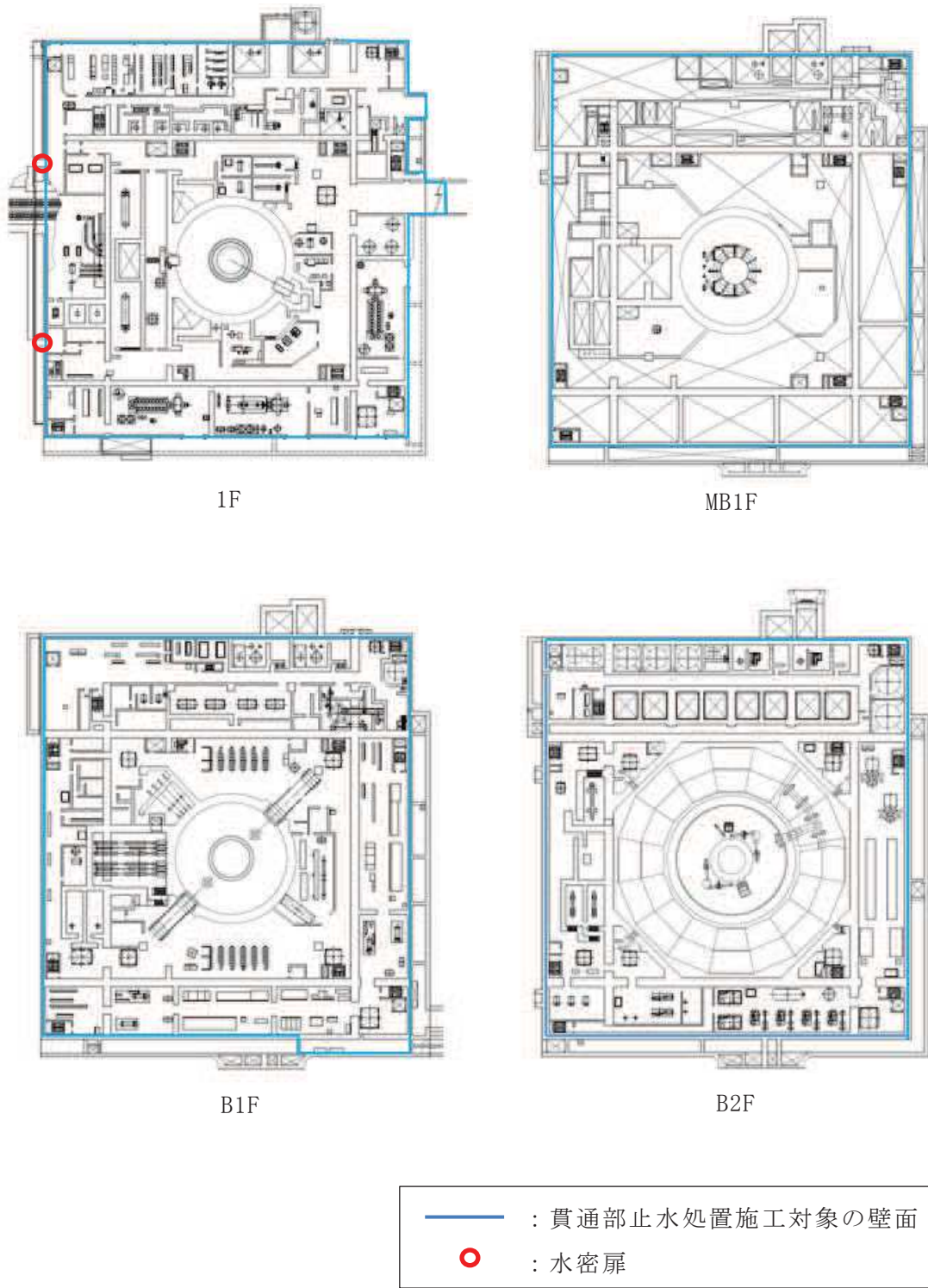
図 3-43 貫通部止水処置及び水密扉の位置図 (2/5) (原子炉建屋)
