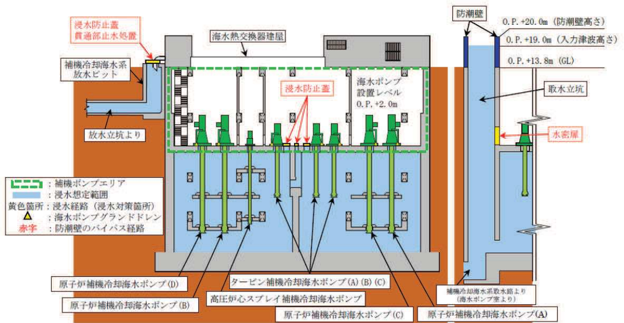
図 2-4 (9) 第 3 号機 海水熱交換器建屋 浸水対策配置図
