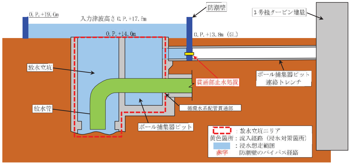
図 2-4 (16) 第 3 号機 放水立坑 浸水対策配置図 (A-A 断面図)
