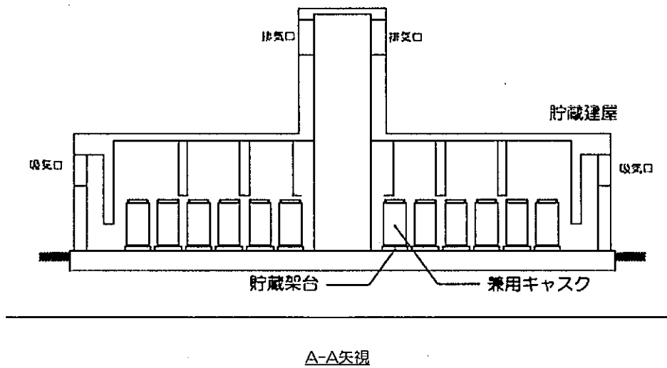
図 1-3 貯蔵施設概要図(例)
