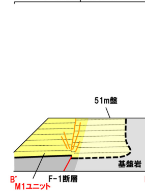
F-1断層開削調査箇所
