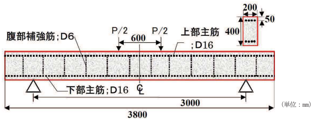
図 3-17 実験概要図
