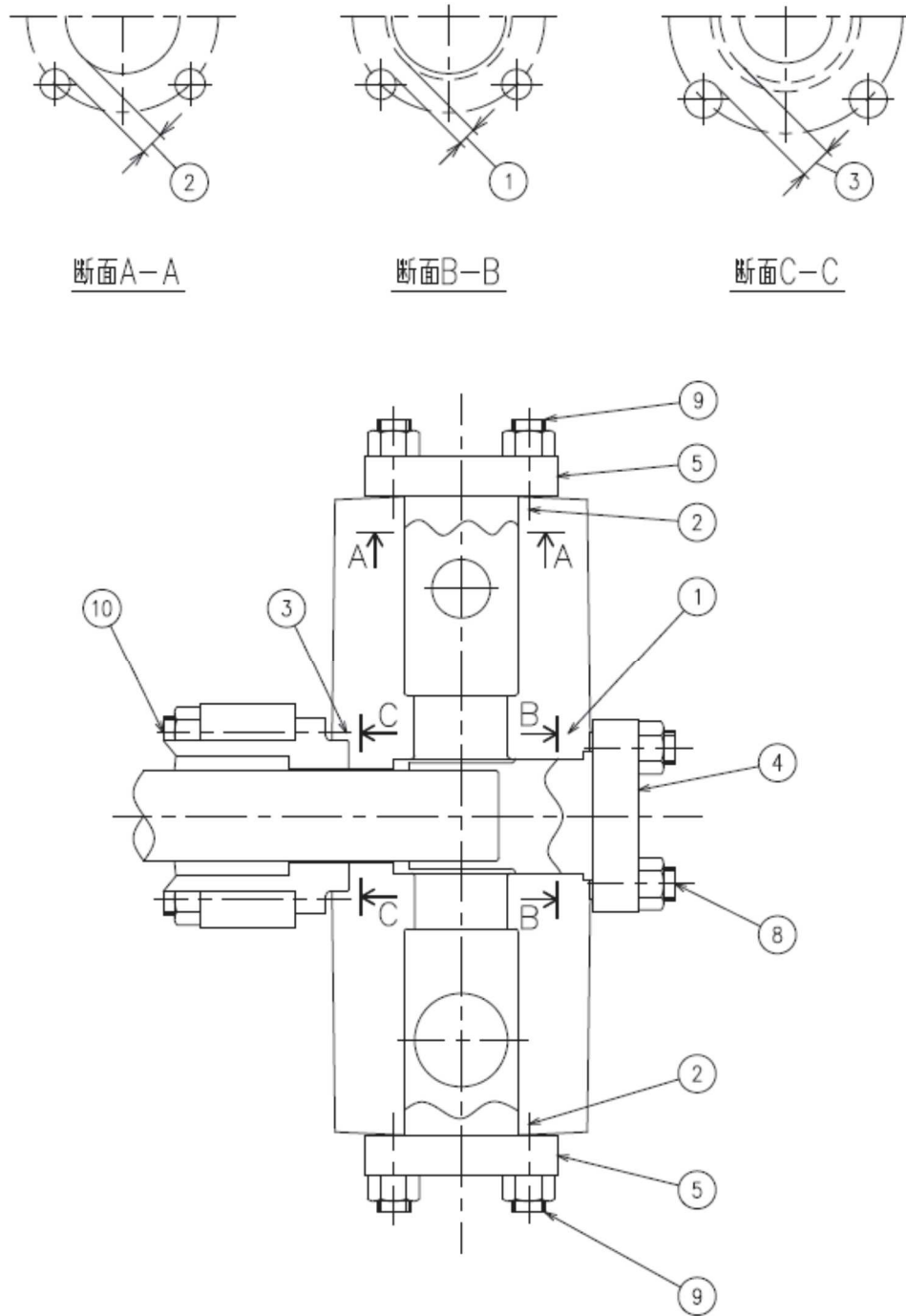
図1-1 概要図 (その1)
