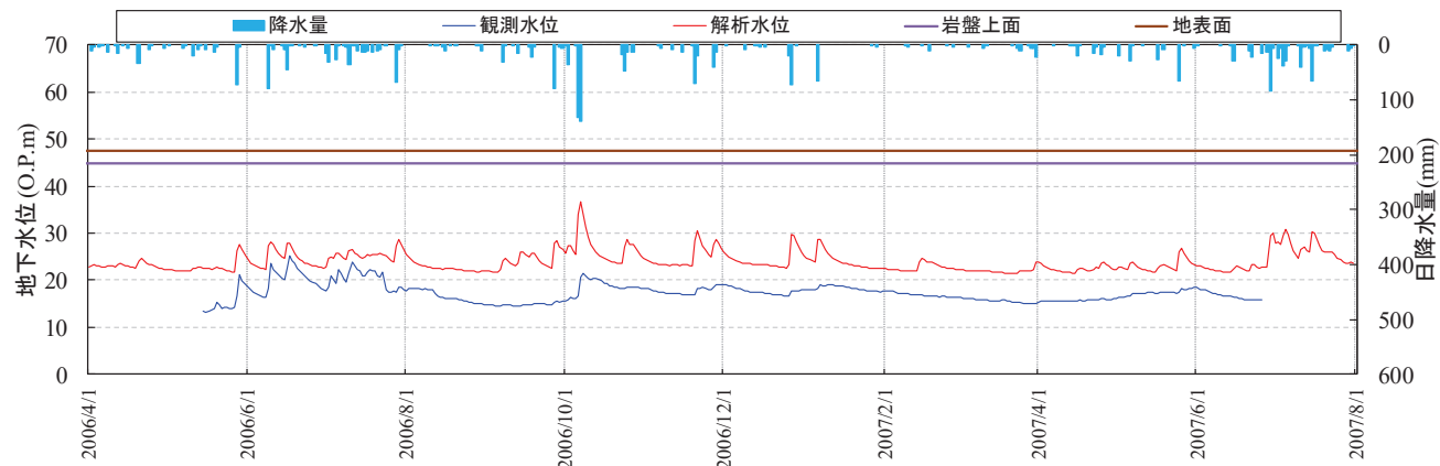
解析水位と観測水位の比較その2(観測井⑩)
