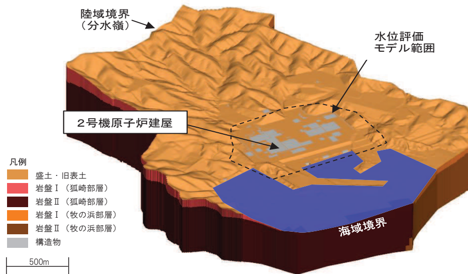
広域モデル鳥瞰図
