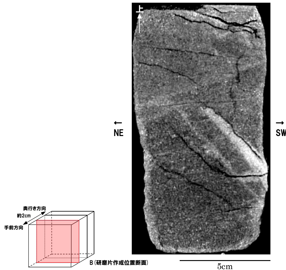
X線CT画像(傾斜方向断面, 解釈線なし) (断面(B):研磨片作成位置断面, P201断面再掲)
