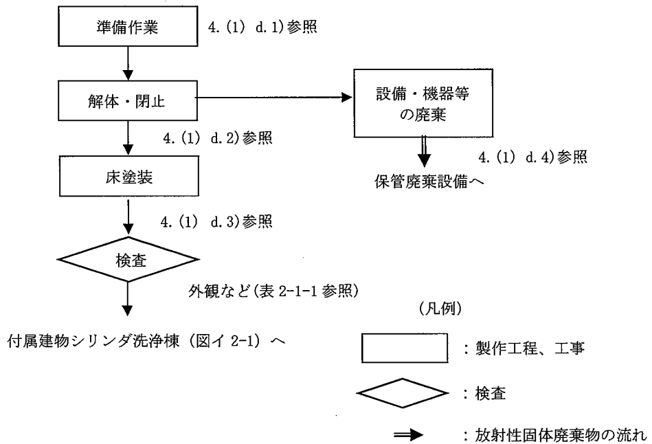
図イ 2-5 工事の手順フロー図 (撤去)
