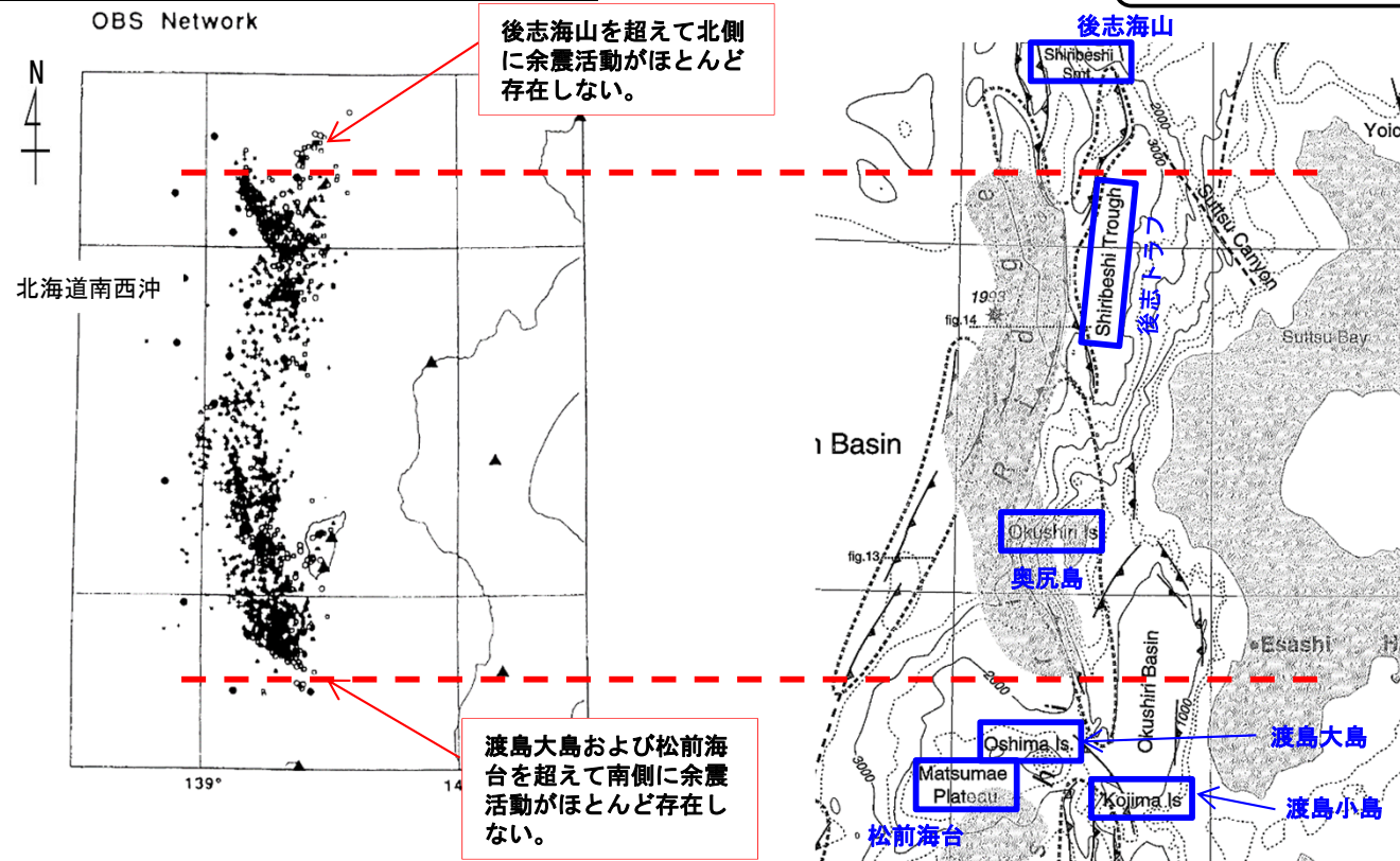
93. 7.21 12:00 - 93. 8.16 23:59 1993年北海道南西沖地震の余震分布
