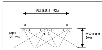
東西方向位置・傾斜角及び傾斜方向パターン 土木学会 (2016) (8) に一部加筆
