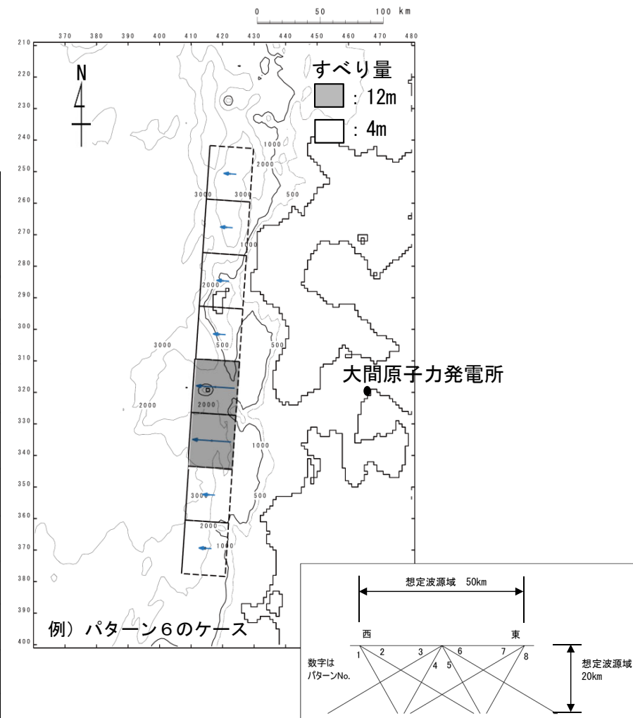
東西位置, 傾斜角パターン 土木学会 (2016) (8) に一部加筆 基準波源モデル
