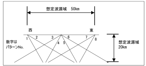
東西位置、傾斜角パターン 土木学会 (2016) (8) に一部加筆
