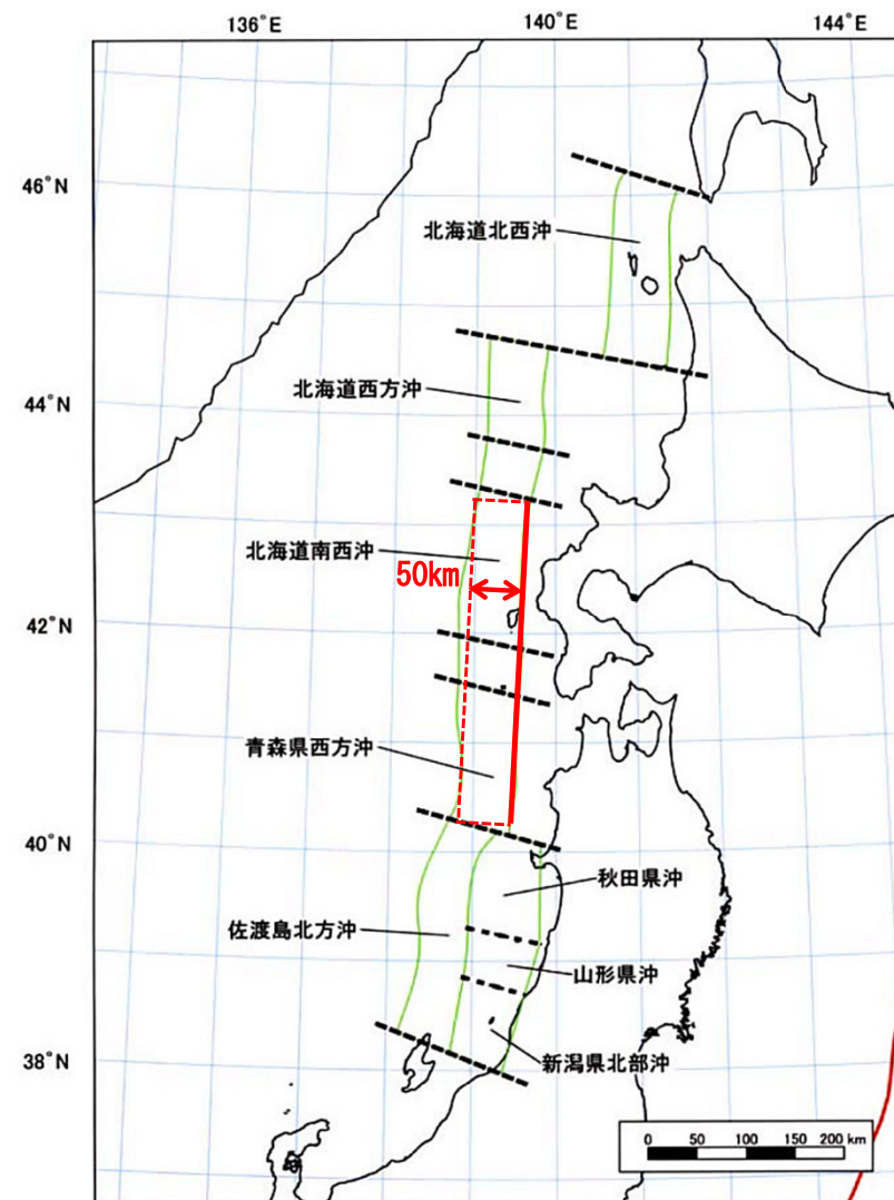
日本海東縁部の想定震源域（東西方向）
