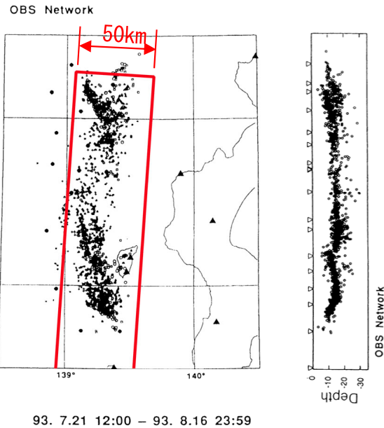
1993年北海道南西沖地震の余震分布
