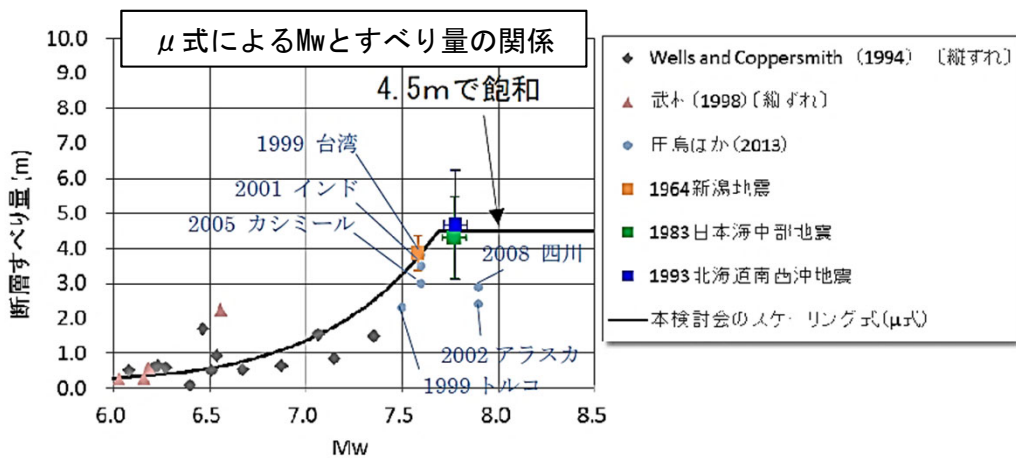
地震規模とすべり量の関係 (日本海における大規模地震に関する調査検討会) 国交省ほか (2014) (2) に一部加筆
