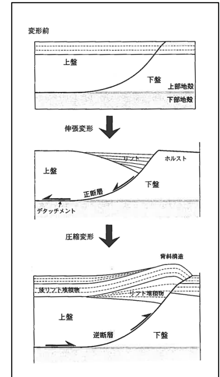
圧縮応力場および伸張応力場で形成される模式的な断層とそれに伴う構造
