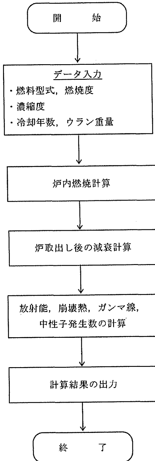
図 2.4.2-9 ORIGEN2 コードの計算フロー図
