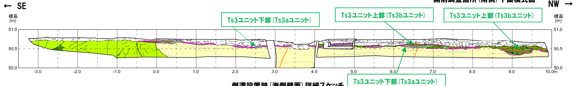
側溝設置跡(海側壁面)詳細スケッチ
