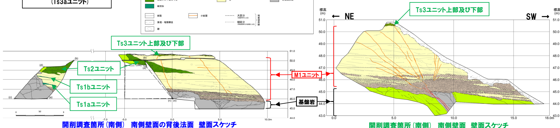
開削調査箇所(南側) 南側壁面の背後法面 壁面スケッチ
