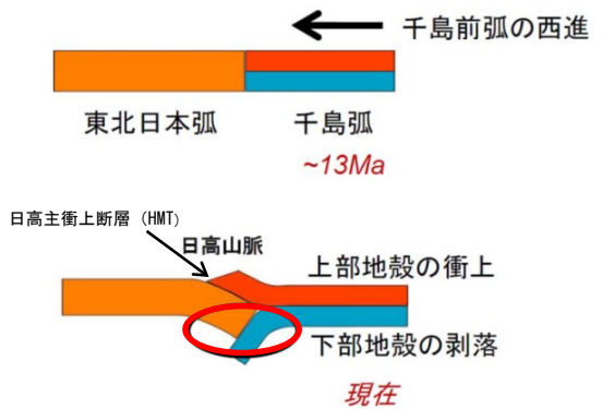
千島弧の前弧スリバーの西進、東北日本弧との衝突による日高山脈形成過程の模式図 日野ほか (2008) (73)に一部加筆
