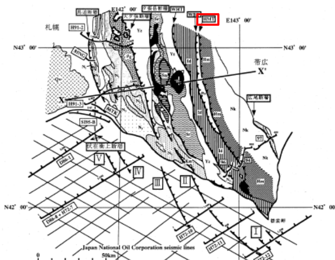
図1 日高山脈帯ならびに前縁褶曲・衝上断層帯の地質概略と主な反射法地震探査測線図。X-X'は図2の断面位置を示す。伊藤ら(1999)を改変。 【地質】主として、地質調査所(1982, 1996)による。Nk: 中の川層群, Hm: 日高変成岩類(主帯), Po: ポロシリ・オフィオライト(西帯), Id: イドンナップ帯, Yz: 蝦夷層群, Sr: 空知層群, Km: 神威古澤変成岩類, Sn: 沙流川層-ニセウ層, Pg: 古第三系, N1~N3: 地質調査所(1982)と同じ。Qv: 第四紀火山岩類。HMT: 日高主衝上断層, WBT: 西縁衝上断層, WHT: 日高西部断層群 【測線】94・96・97: 日高深部構造反射法探査, 85NG・86TK: 浅野ら(1990), Y97: 佐藤ら(1998), その他の測線は石油公団(1973, 1987, 1993, 1996)。
