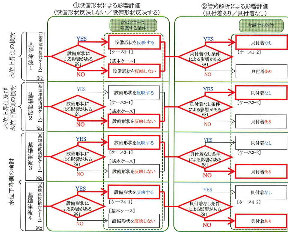
第4-6図 管路解析の影響評価結果
