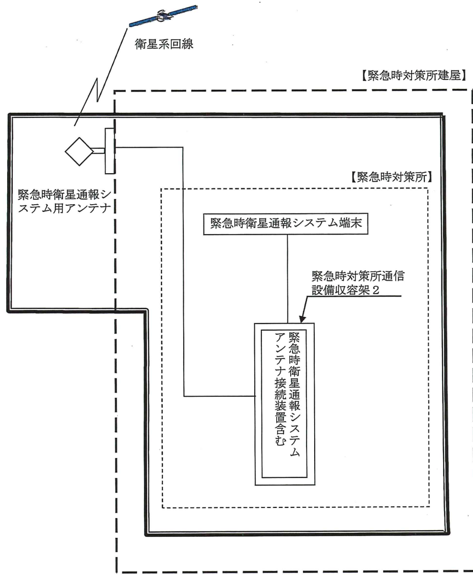
第5図 緊急時衛星通報システム概略構成図
