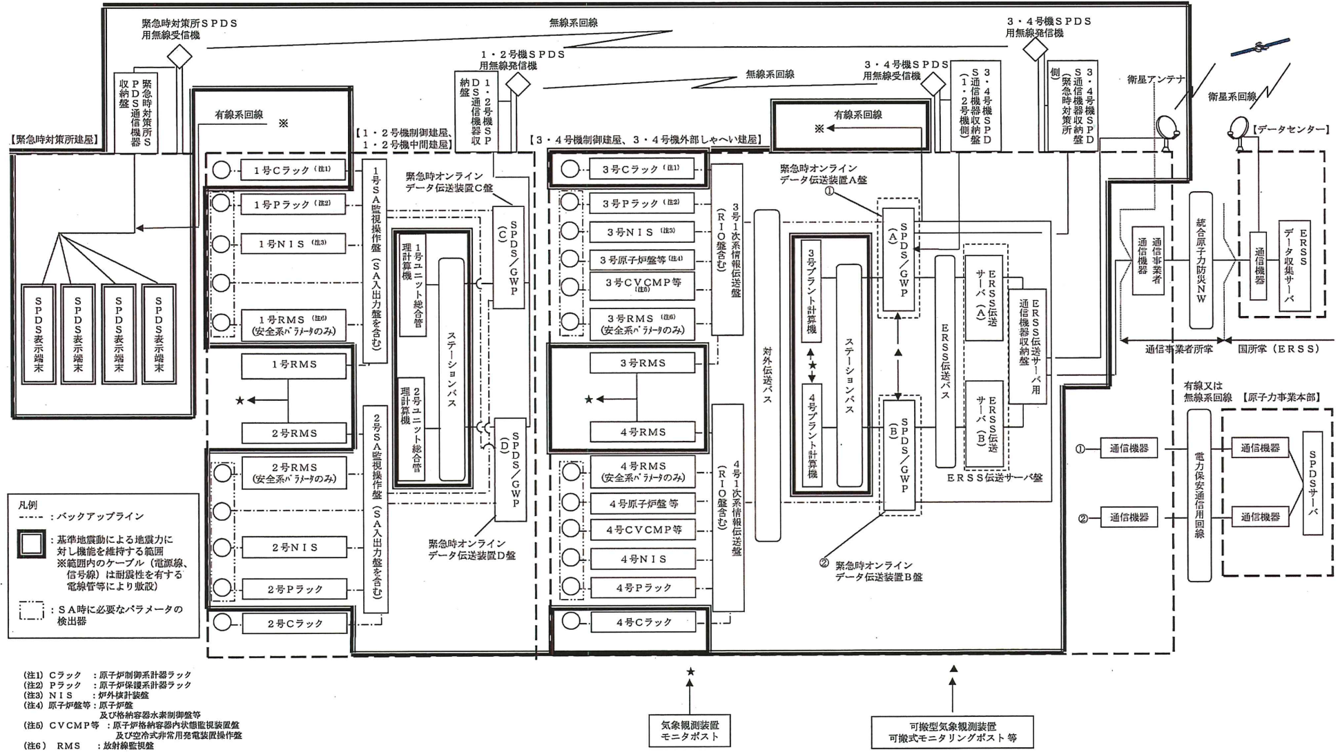
第3図 データ伝送設備の概略構成図
