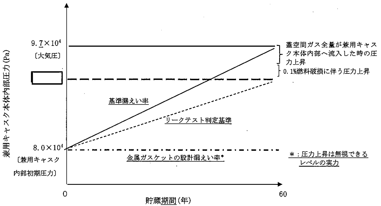
図 2.4.4-5 兼用キャスク漏えい率の考え方
