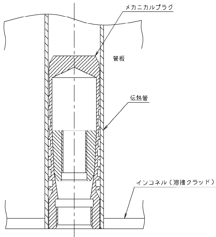
メカニカルプラグ取付図
