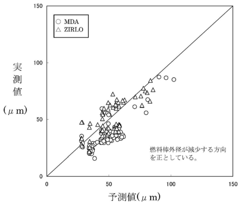
第3-7図 MDA及びZIRLO被覆管外径変化(クリープダウン)の実測値と予測値の比較 (13)(14)
