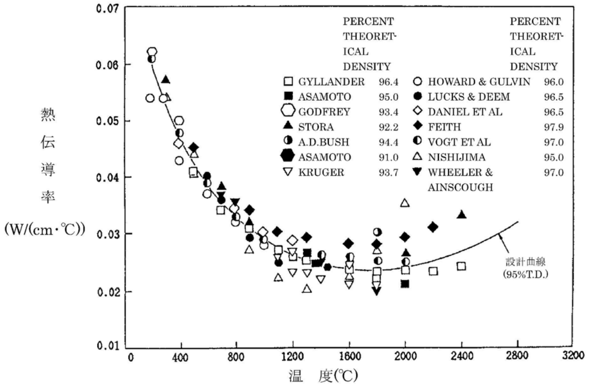
第3-8図 二酸化ウランの熱伝導率 (図中のプロット点は全て95%T.D.に補正後の値を示す。)
