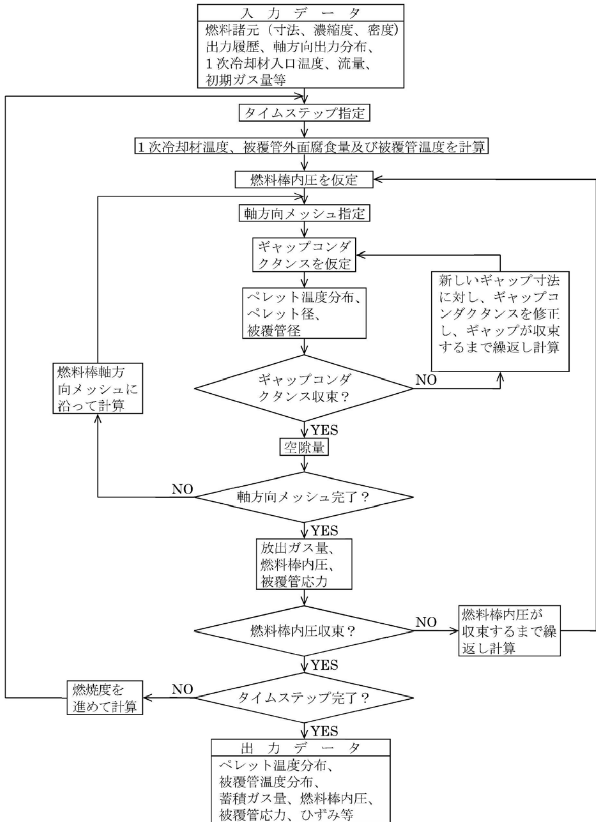
第3-2図 高燃焼度用 FINE コードのフロー図
