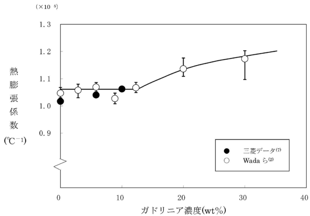
第3-4図 ガドリニア入り二酸化ウランペレットの熱膨張係数 (2)(7)
