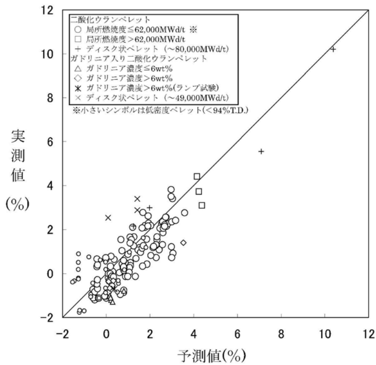
第3-5図 ペレット体積変化の実測値と予測値の比較 (8)(9)(10)
