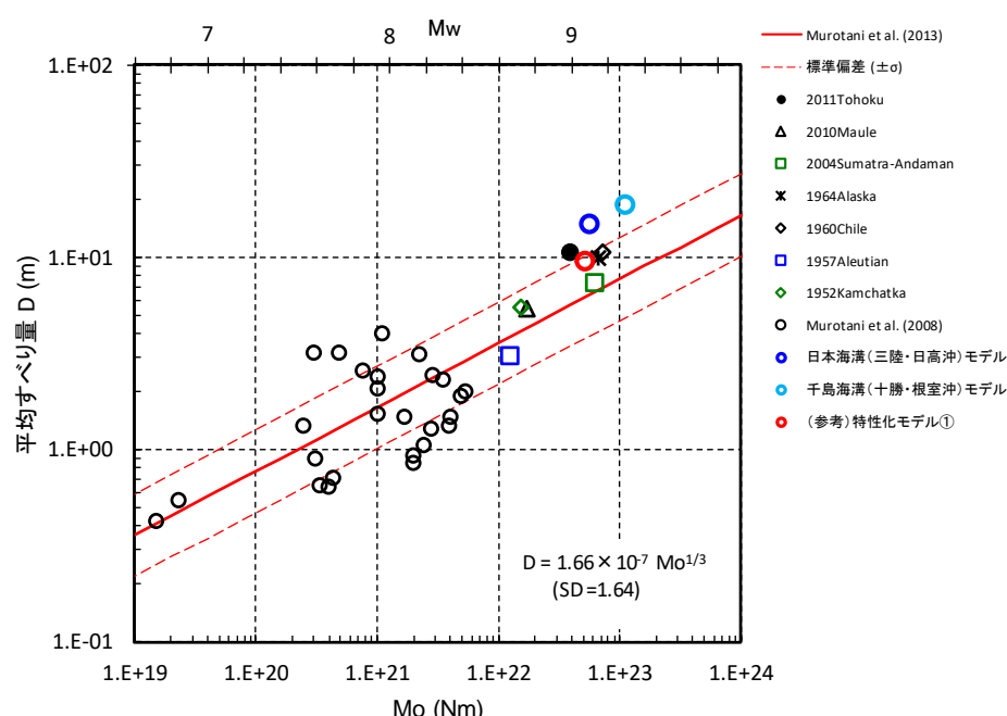
平均すべり量(D)とM 0 の関係 (Murotani et al.(2013)一部修正・加筆)
