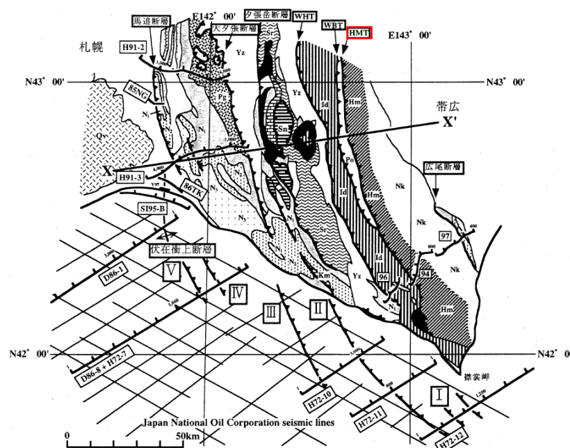
図1 日高衝突帯ならびに前縁褶曲・衝上断層帯の地質概略と主な反射法地震探査測線図。X-X'は図2の断面位置を示す。伊藤ら(1999)を改変。
