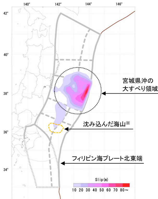
3.11地震時のすべり量分布
