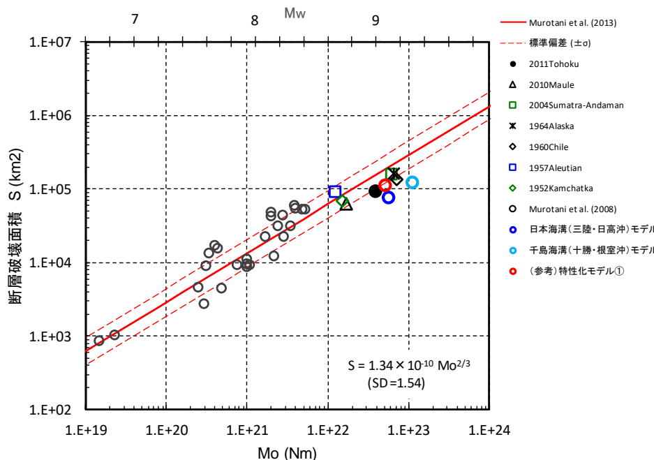
破壊領域(S)とM 0 の関係 (Murotani et al.(2013)一部修正・加筆)
