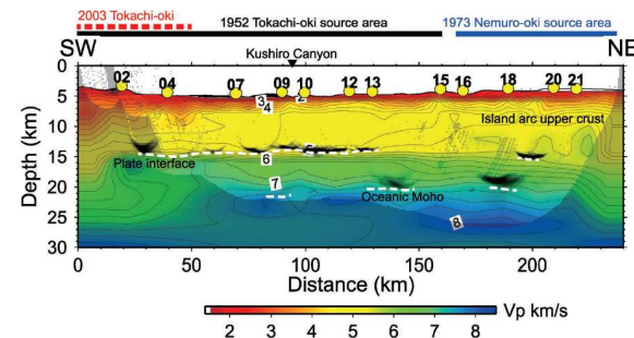
十勝沖・根室沖におけるアスペリティと 2003年十勝沖～1973年根室沖の震源 域間のP波速度構造(2010年測線) (東(2012))
