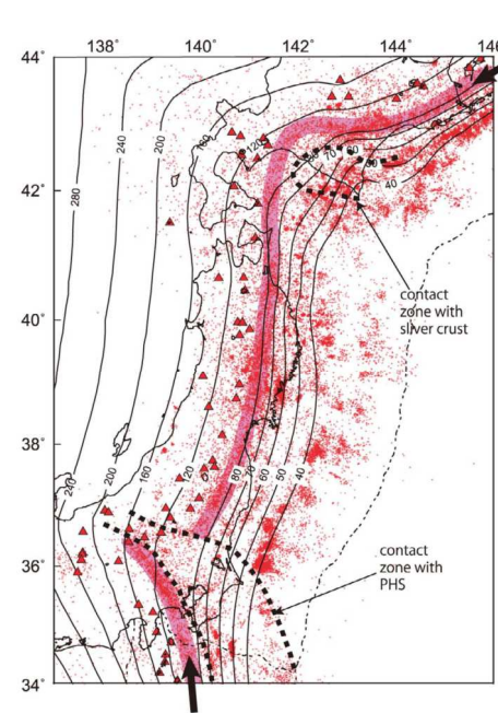
太平洋スラブ地殻内の地震の分布 (長谷川ほか(2012)) 赤点:プレート境界から下方に0~10kmの範囲の地震 ピンク色の網目:上面地震帯 黒線:太平洋スラブ上部境界面の形状 黒点線:太平洋スラブが直上のフィリピン海スラブ及び前弧スリバー地殻と接触している領域
