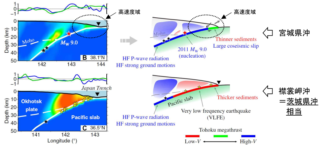
プレート境界におけるP波速度分布とそのイメージ(p159再掲) (Liu and Zhao(2018)に一部加筆)
