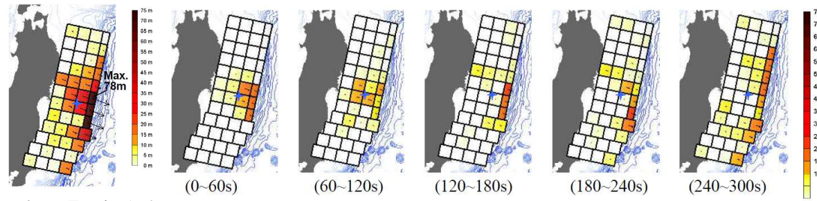
すべり量の時間変化(確定波源モデル)
