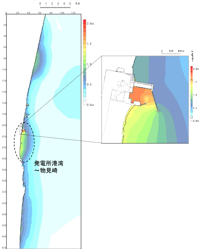
■ 発電所港湾～物見崎 (入射波周期: 12分)
