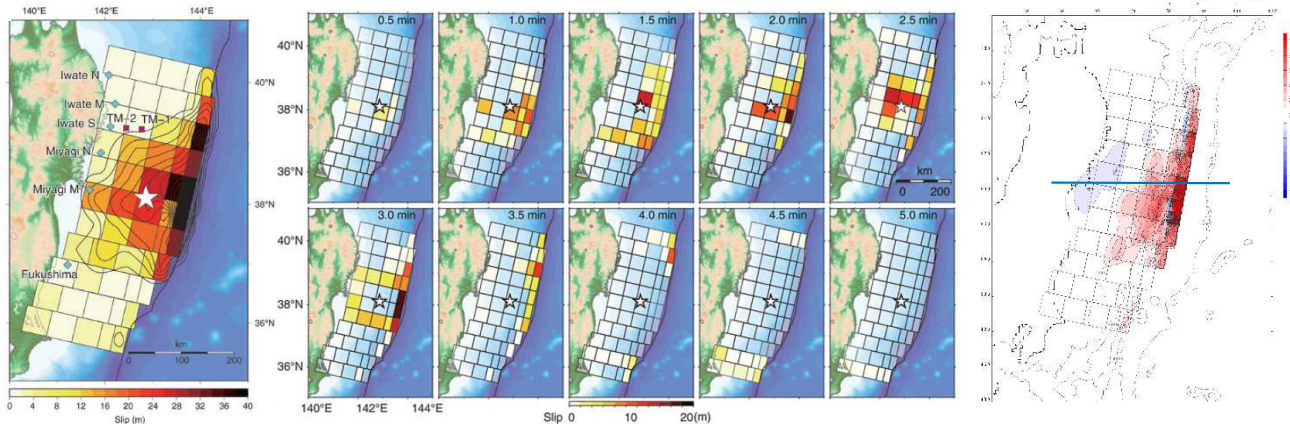
地殻変動量分布(合計)
