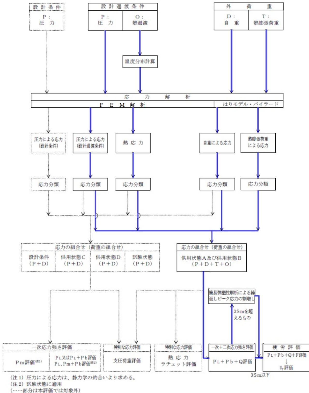
応力評価フローチャート
