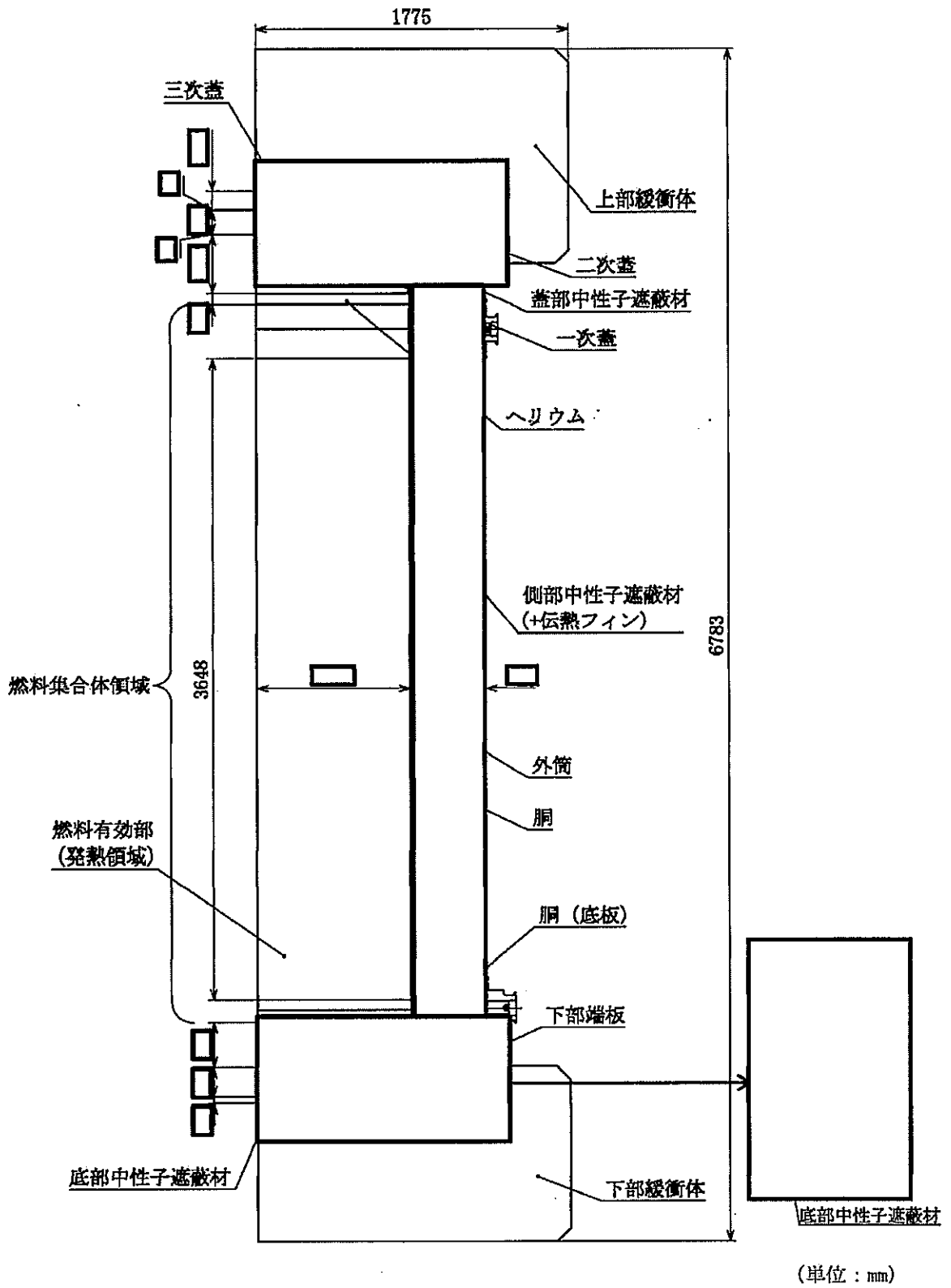
(a)-第 B.1 図 一般の試験条件の全体モデル形状図 (1/2) (縦断面図)
