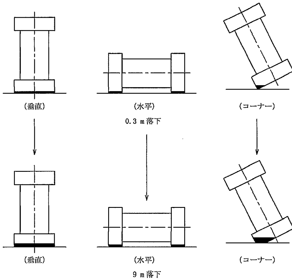
(a)-第 A. 46 図 落下姿勢と試験の順序
