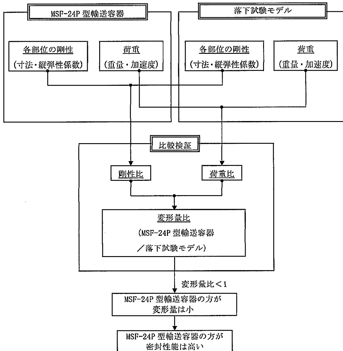
(u)-第 A. 59 図 密封性能評価手順
