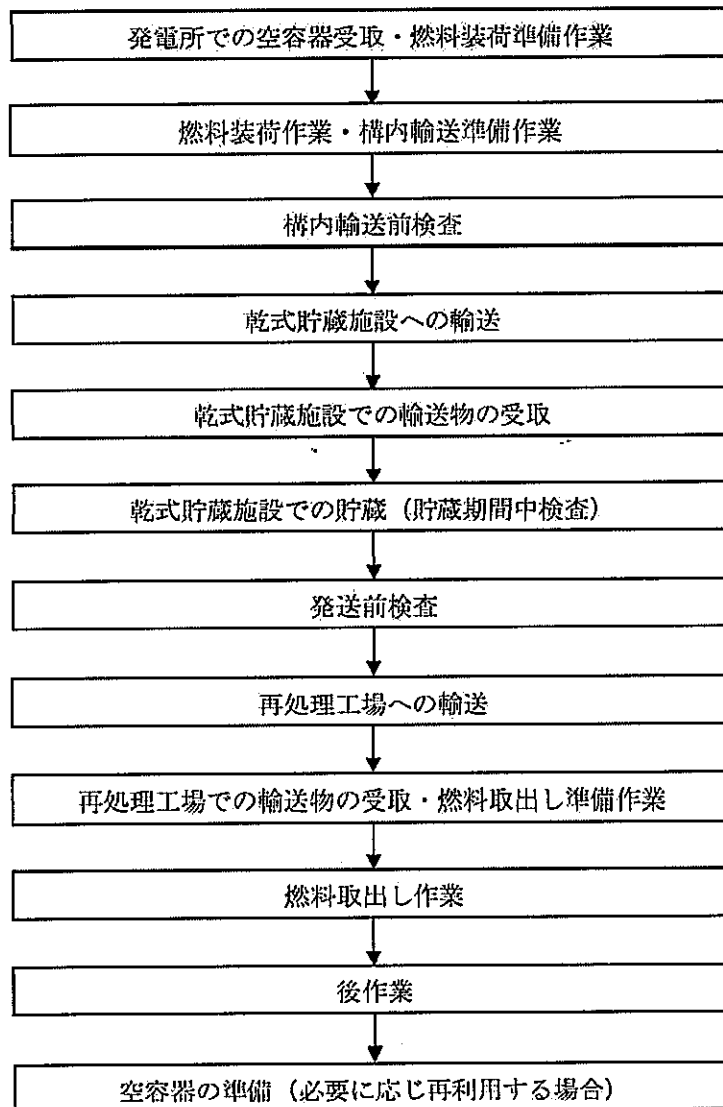
(E)-第 A.1 図 標準的な輸送物の取扱いの流れ
