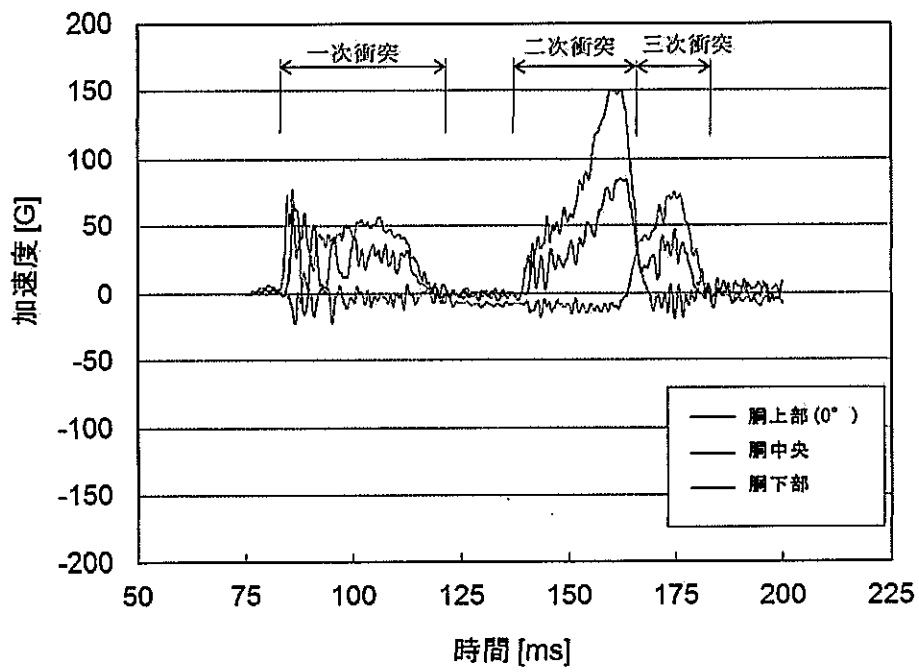
(ア)-第 A. 56 図 9.3 m 傾斜落下時の落下方向加速度履歴
