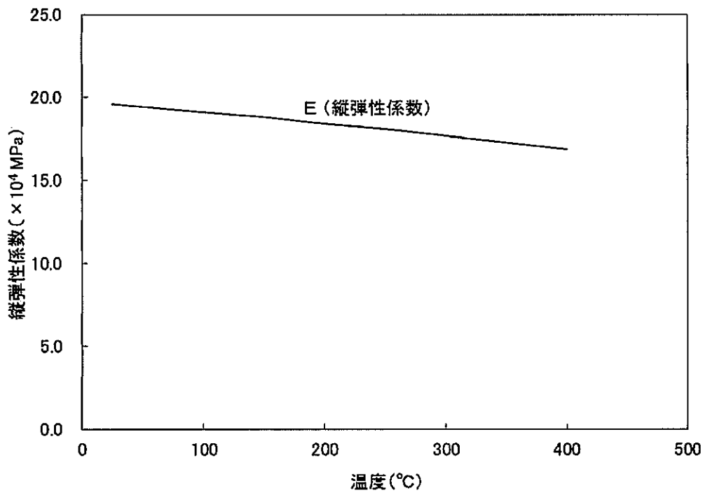
(p)-第 A. 5 図 析出硬化系ステンレス鋼 (SUS630-H1150) の 温度に対する機械的性質の変化 (2/2) 1), 3)
