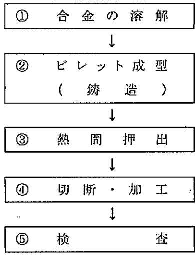
(ア)-第A.63図 製造フロー
