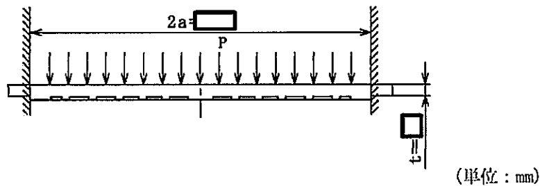
(Ⅱ)-第 A.45 図 外圧に対する三次蓋の解析モデル
