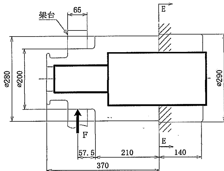
(a)-第 A. 14 図 輸送架台固縛状態解析モデル図
