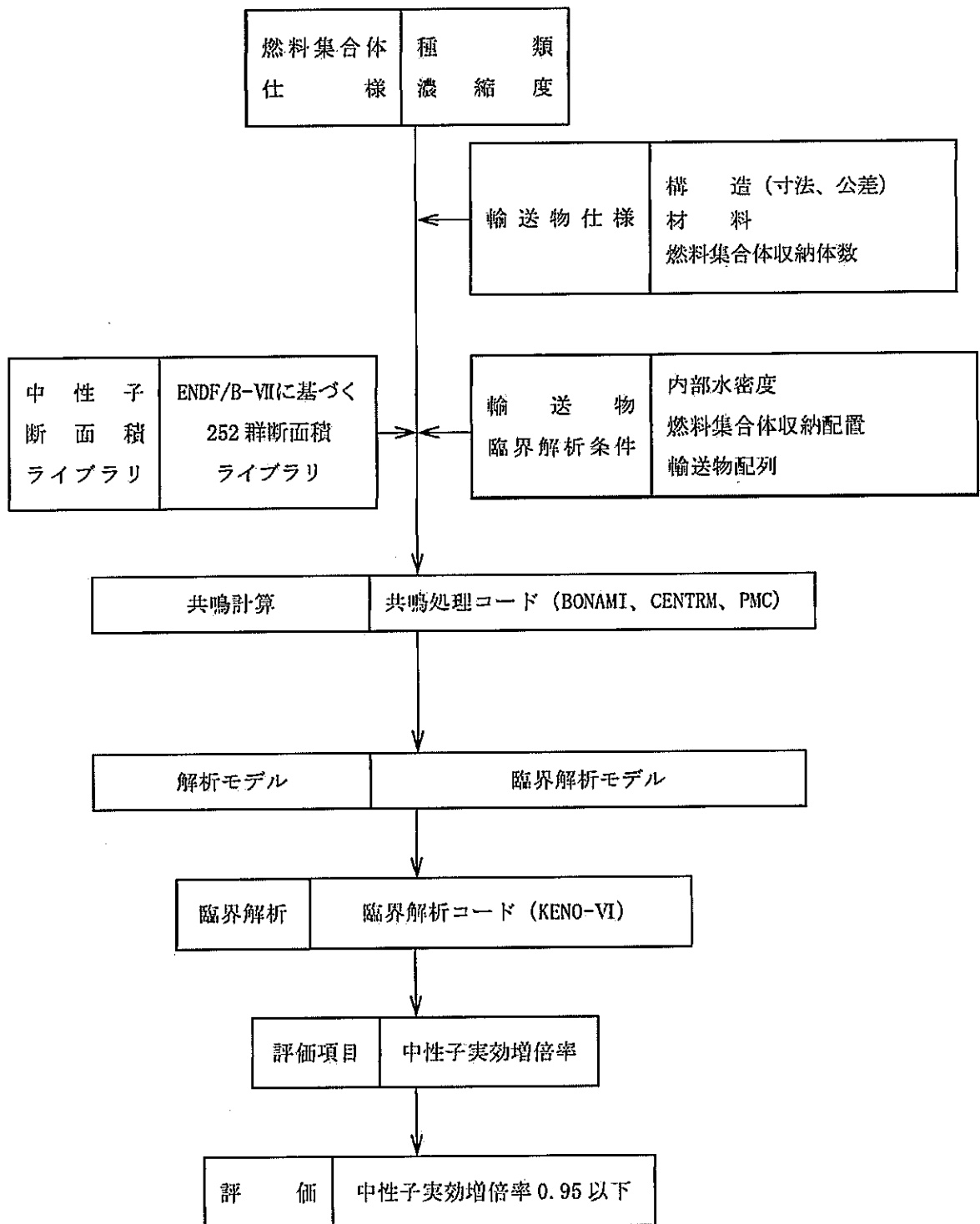
(p)-第 E.3 図 臨界計算の流れ
