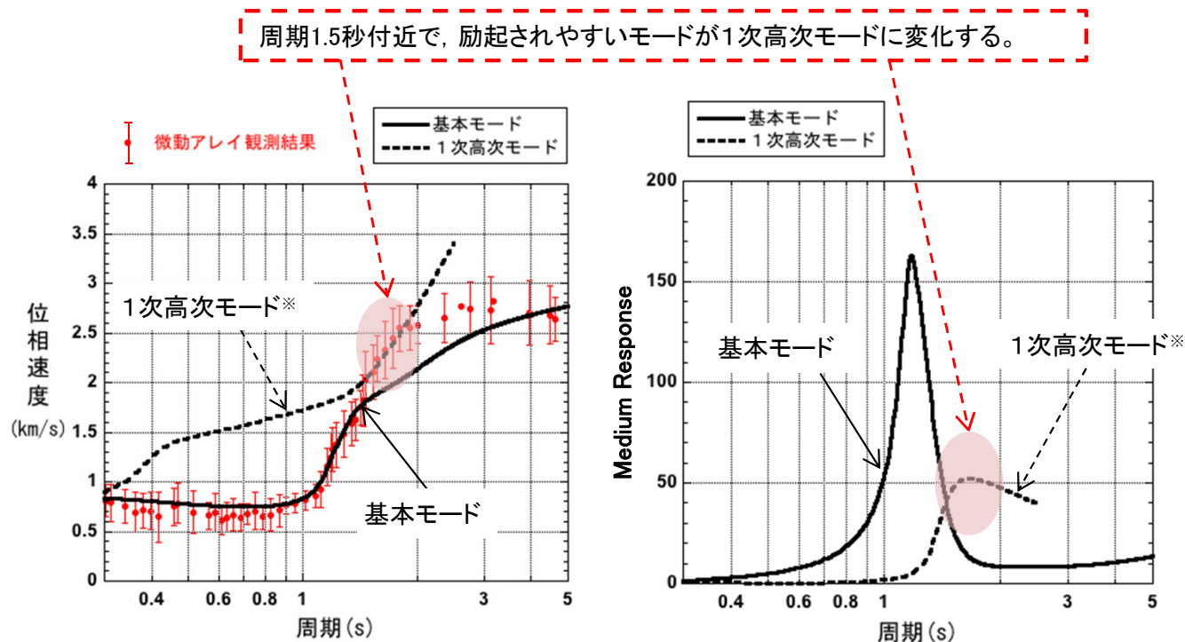
最適化地盤モデルの理論分散曲線 と微動アレイ観測結果との比較
