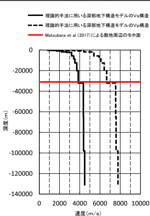
理論的手法に用いる深部地下構造モデルの速度構造と Matsubara et al.(2017)によるモホ面の深さとの関係
