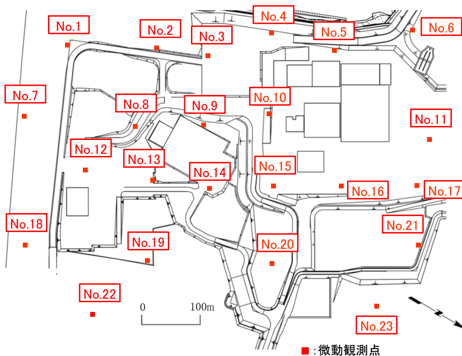
平面アレイ微動観測点
