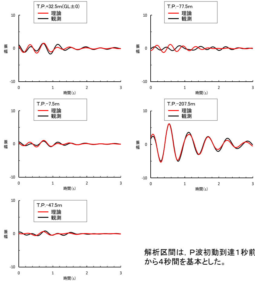
P波部レシーバ関数の比較※
