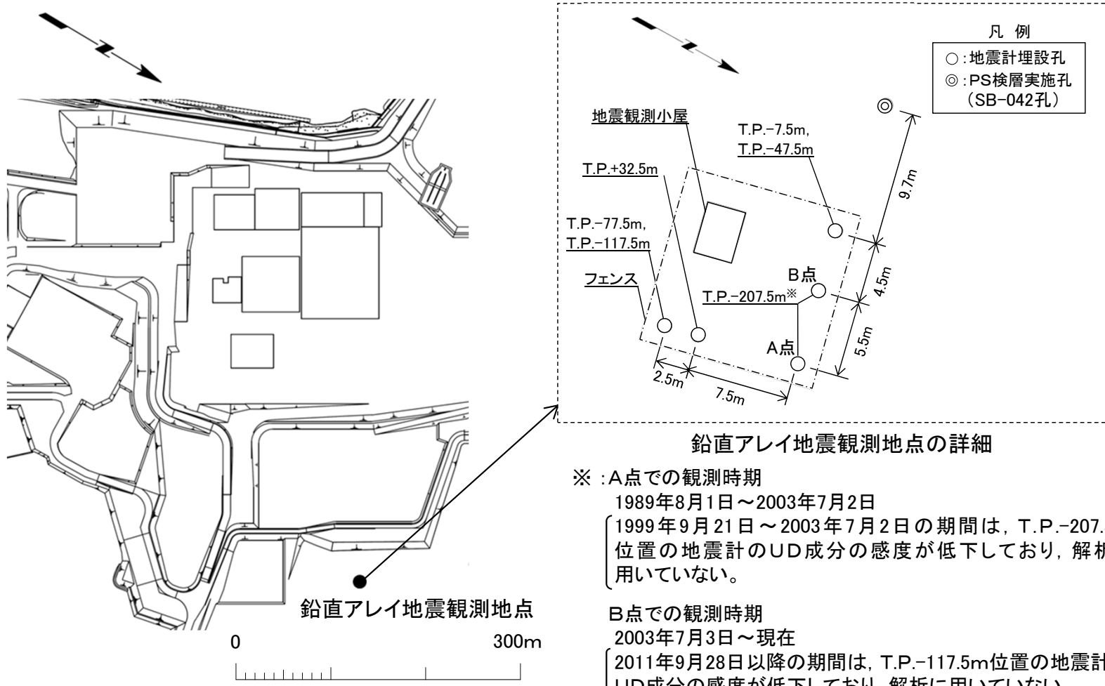
鉛直アレイ地震観測地点の位置
