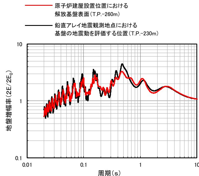
図2 原子炉建屋設置位置における解放基盤表面及び鉛直アレイ地震観測地点における基盤の地震動を評価する位置の地盤増幅率の比較※3 (評価位置の 2E/ 地震基盤位置の入力波 2E_0 )
