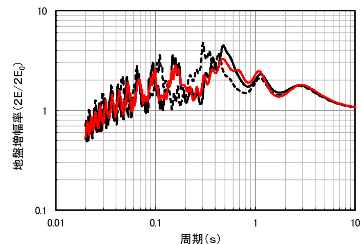
図2 原子炉建屋設置位置における解放基盤表面及び鉛直アレイ地震観測地点における基盤の地震動を評価する位置の地盤増幅率の比較 (評価位置の 2E /地震基盤位置の入力波 2E_0 )
