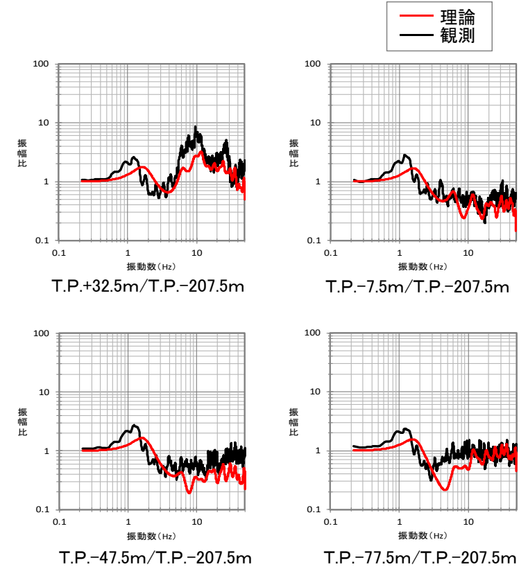
最適化地盤モデルの理論伝達関数と観測記録に基づく伝達関数の比較
