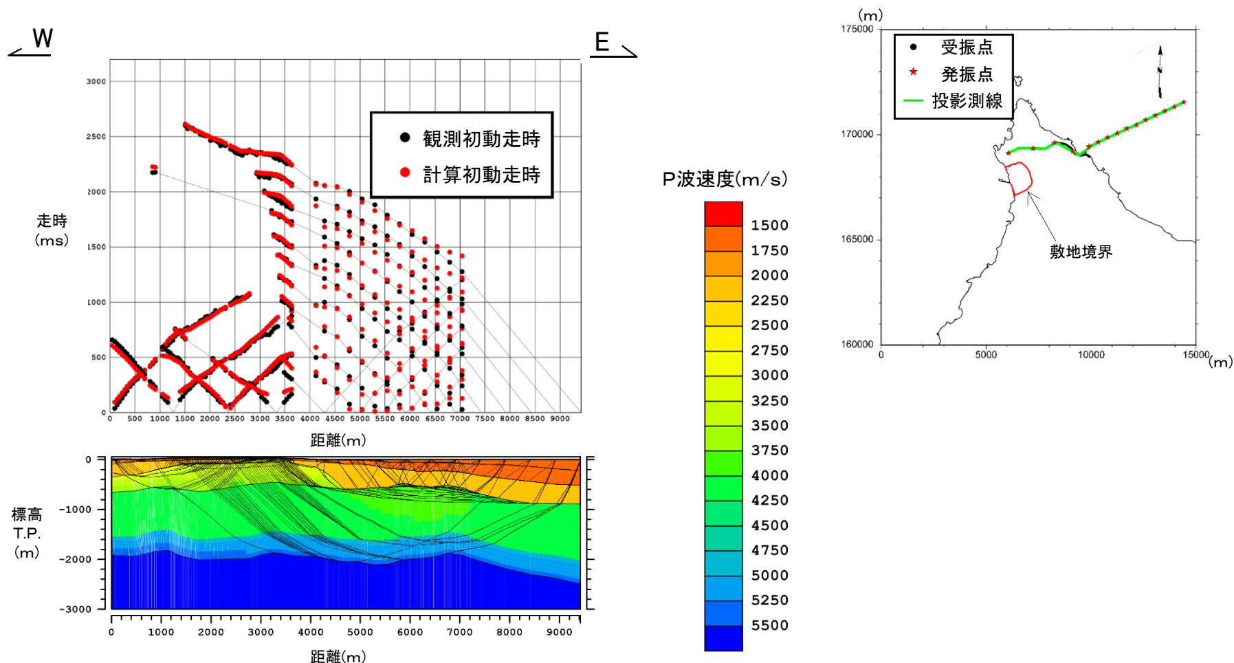
陸海連続弾性波探査の再現解析結果
