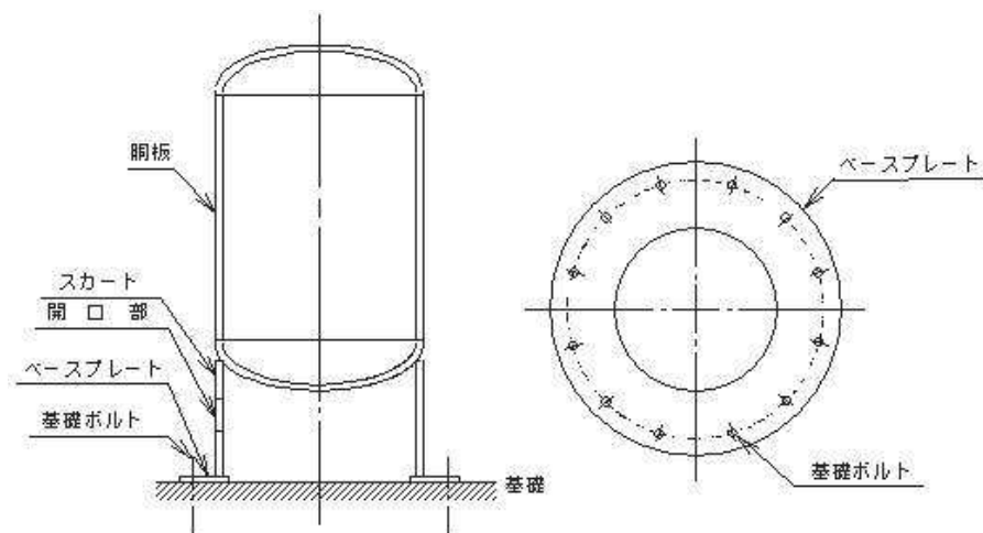
図5-1 概要図
