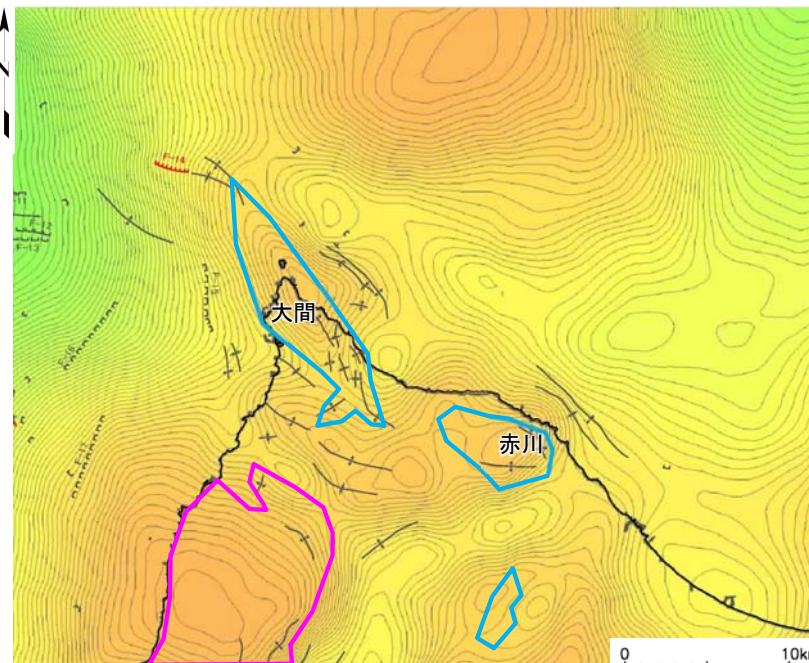
ブーゲー重力異常図
