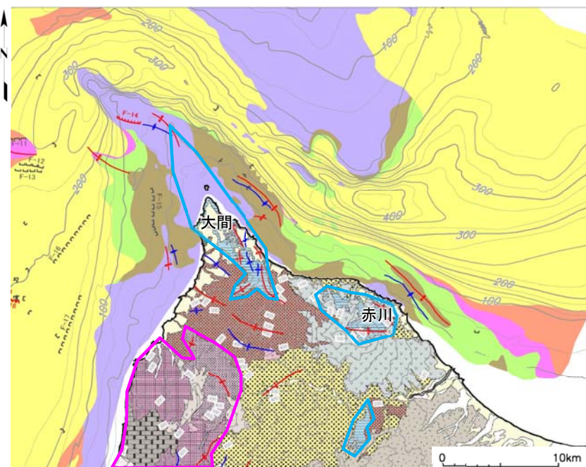
陸域及び海域の地質平面図
