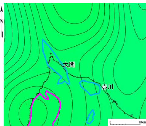
残差重力(10-20km)
