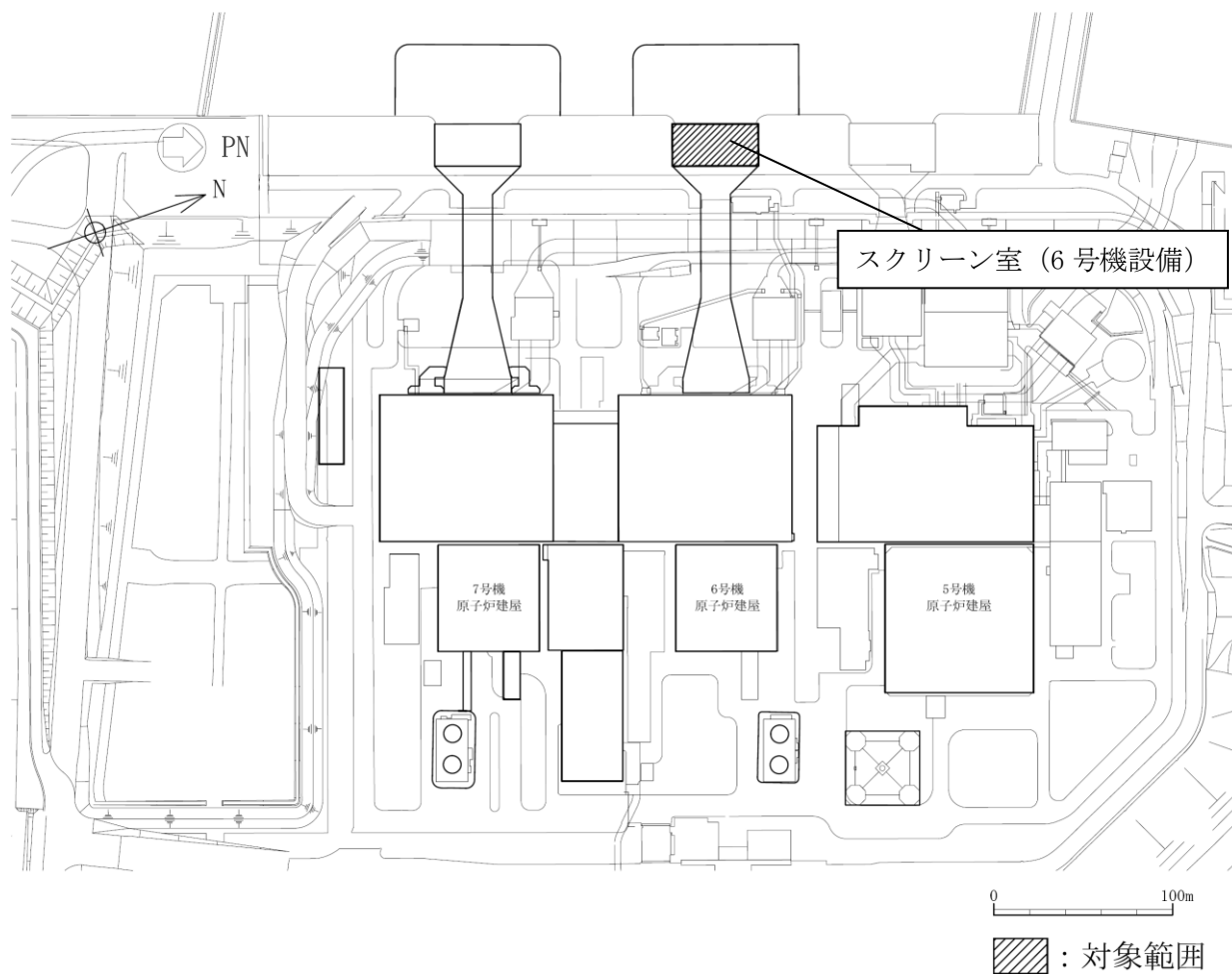
図2-1 スクリーン室（6号機設備）の位置図（全体平面図）
