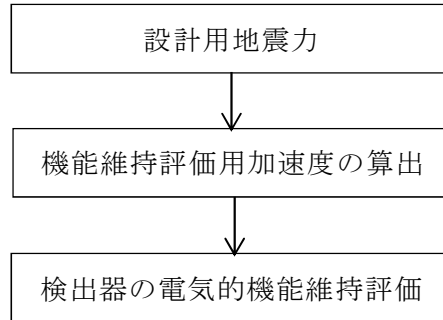
図2-1 残留熱除去系熱交換器入口温度の耐震評価フロー
