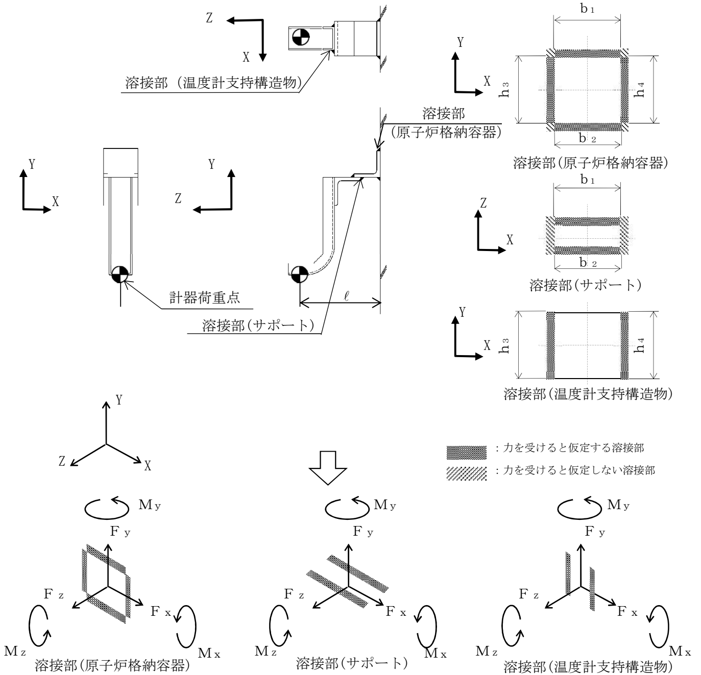
図 2-3 計算モデル (溶接部)
