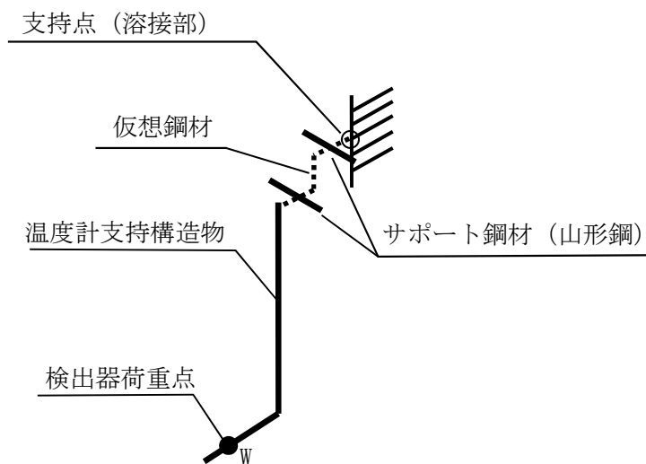
図 2-2 解析モデル
