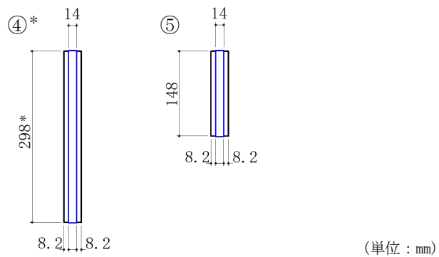
図 2.1-3-31 照査モデル図 (リブプレートと鋼管矢板又は前面鋼矢板接合部)
