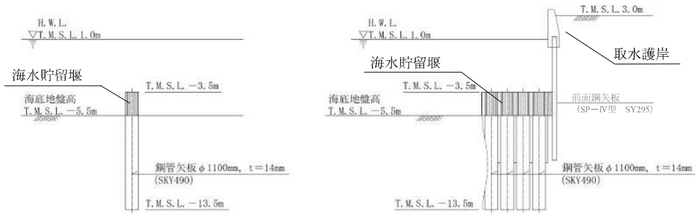
(b) A-A断面図
