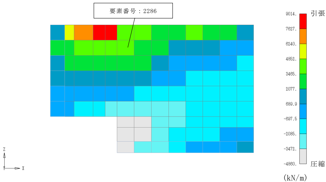
(a) 軸力 (水平方向, ケース 1-8)
