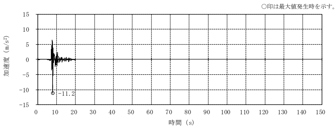
(a) NS方向 並進成分
