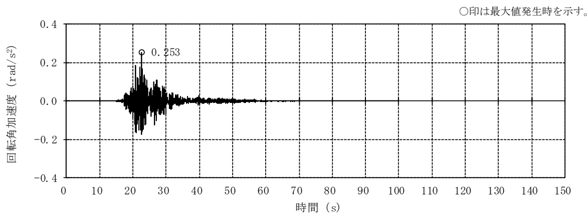
(d) EW方向 回轉成分
