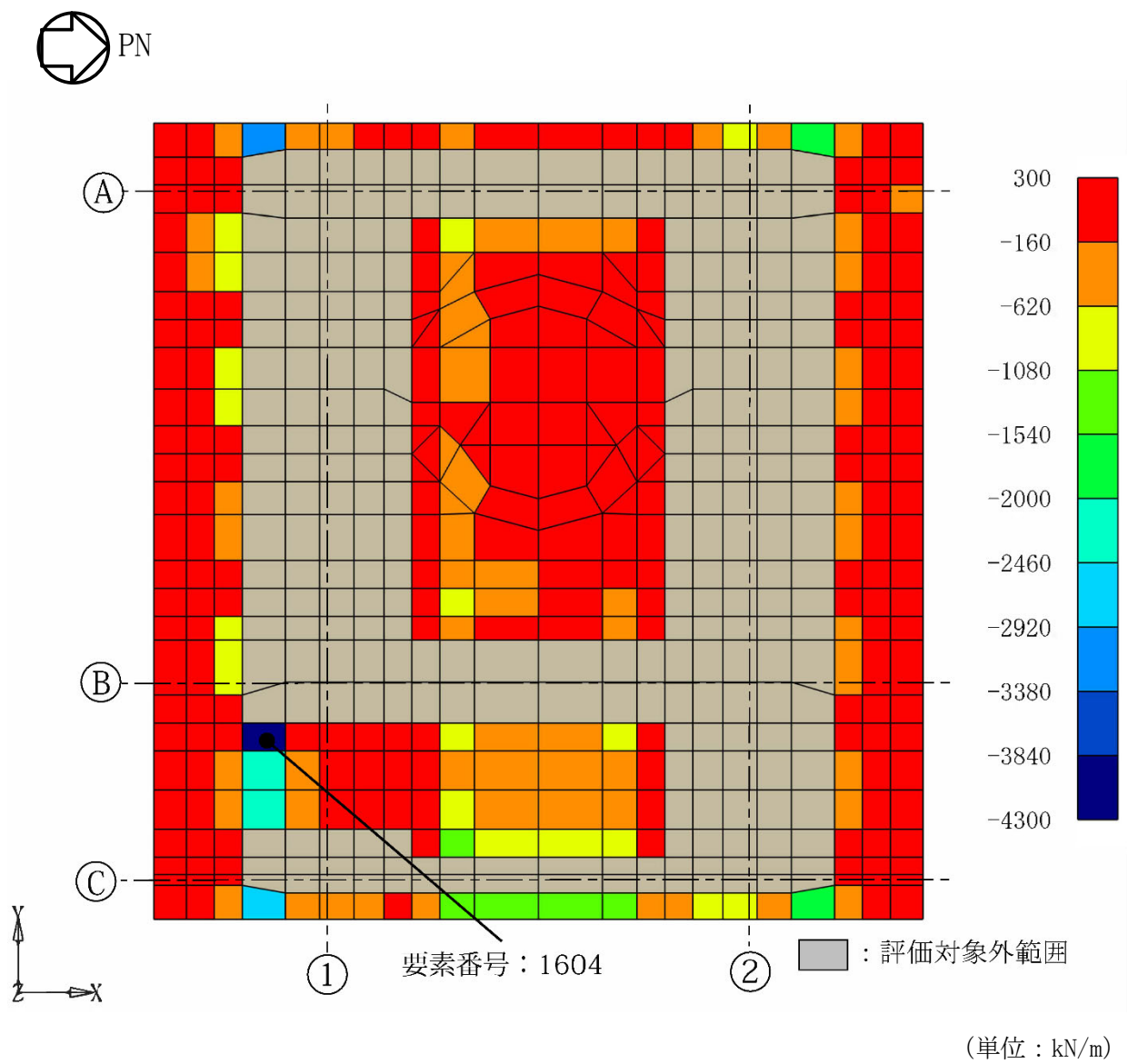
面外せん断力 (NS 方向, ケース 24)
