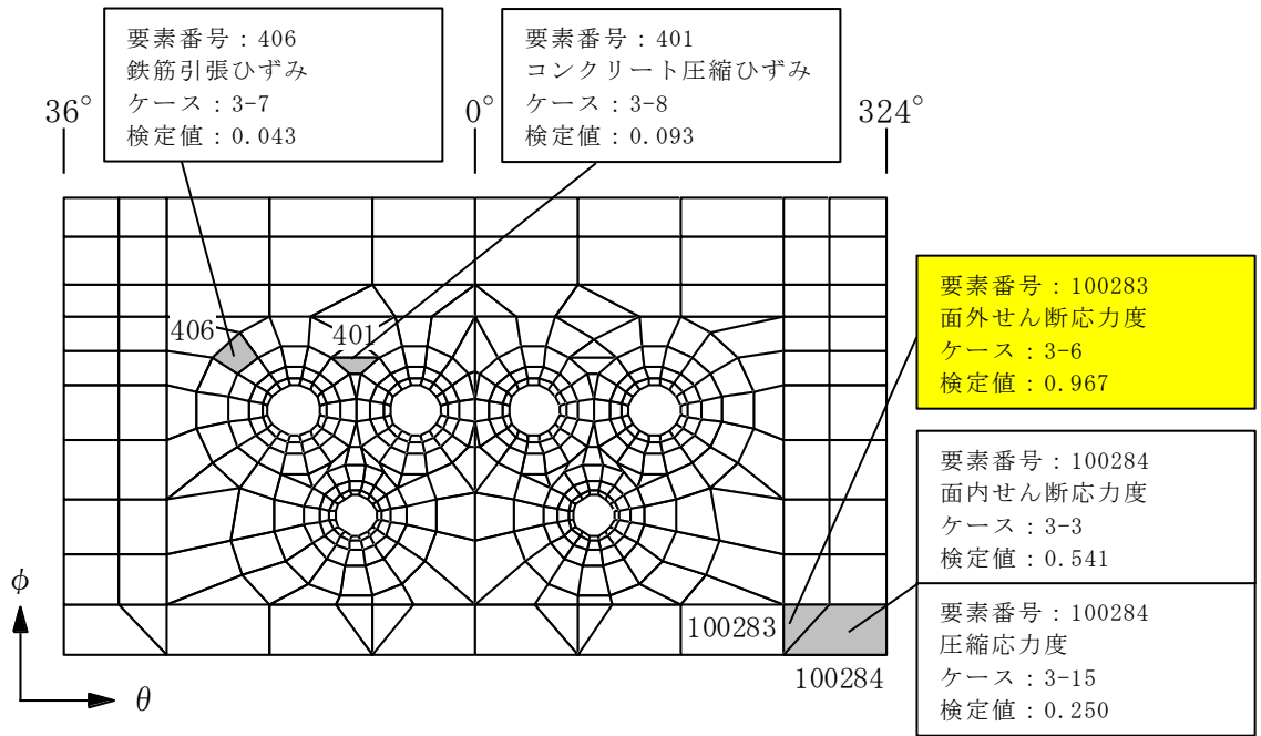
(c) 荷重状態IV・地震時 (2)
