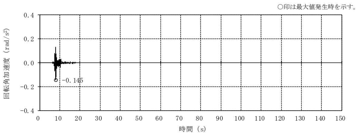
(b) NS方向 回転成分
