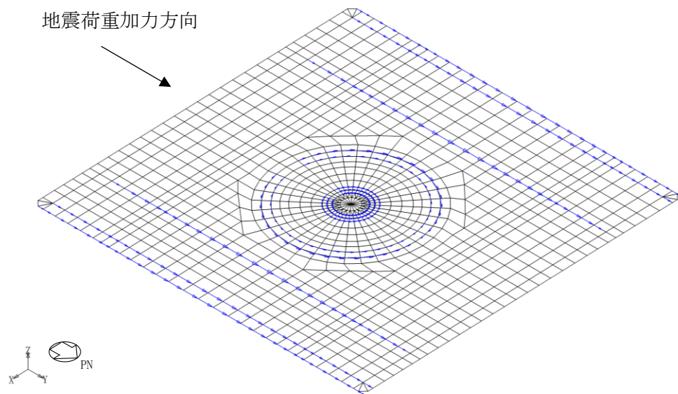
(a) せん断力 (NS 方向) 耐震壁
