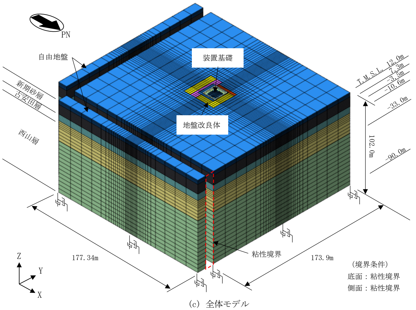
図 2-1 解析モデル
