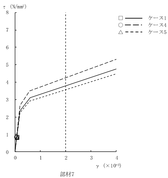
図 2-127 τ - γ 関係と最大応答値 (Ss-3, EW 方向, B1F) (2/4)
