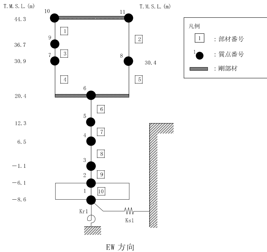
図 5-1 地震応答解析モデル (水平方向)
