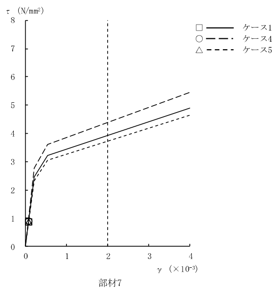
図 2-122 τ - γ 関係と最大応答値 (Ss-2, NS 方向, B1F) (2/4)
