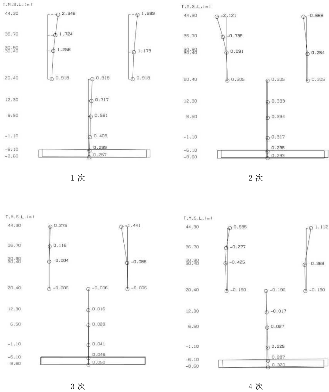
図 4-28 刺激関数図 (ケース 5) (NS 方向, Ss-1) (1/2)
