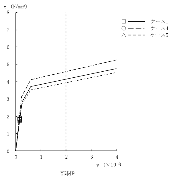
図 2-123 τ - γ 関係と最大応答値 (Ss-3, NS 方向, B3F) (4/4)
