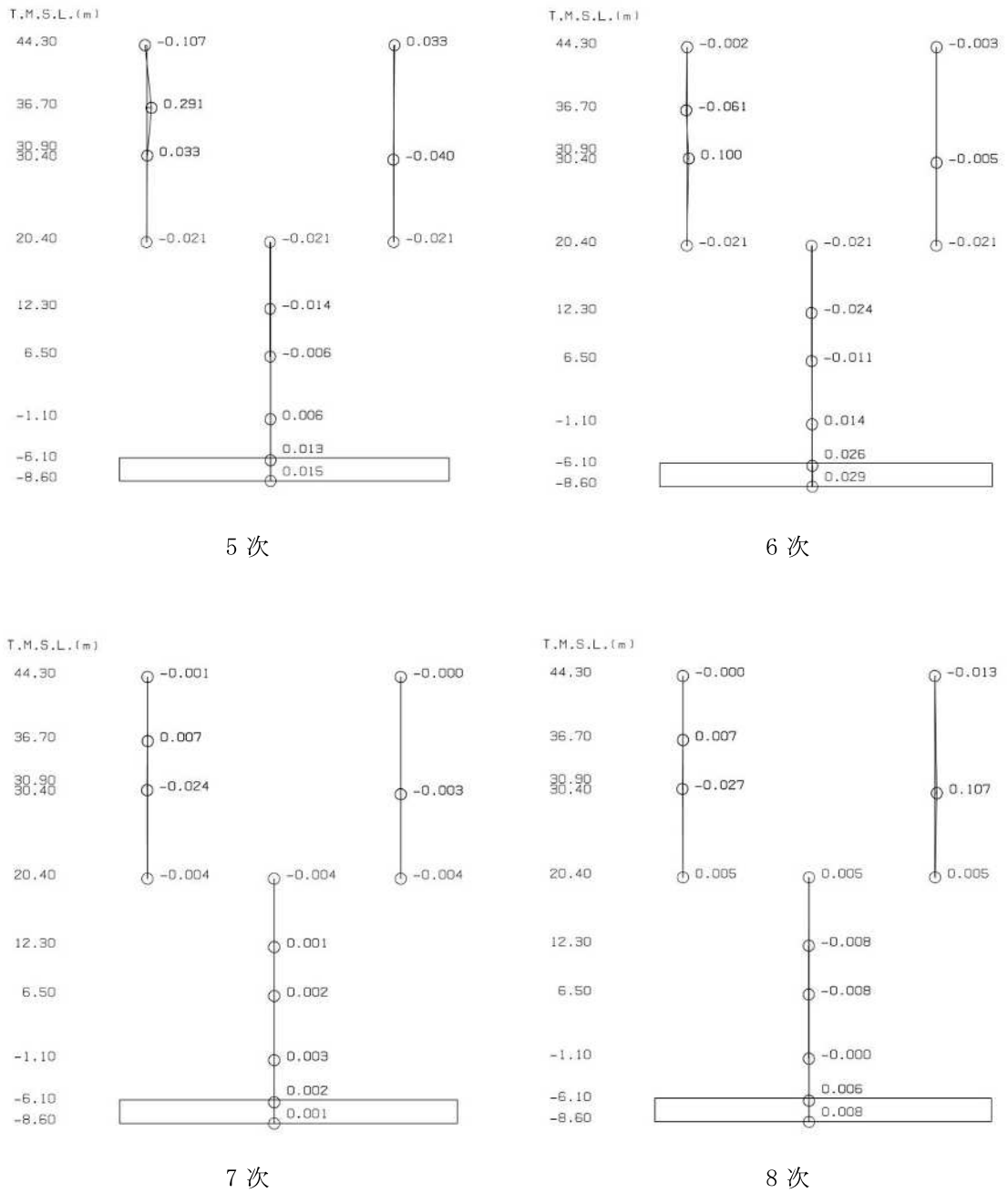
図 4-3 刺激関数図 (ケース 2) (NS 方向, Ss-1) (2/2)
