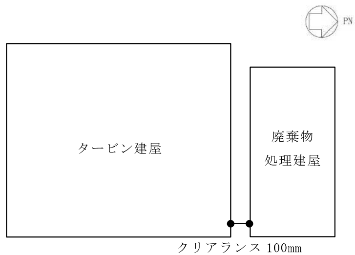
図2-1 建屋配置図（概略図）
