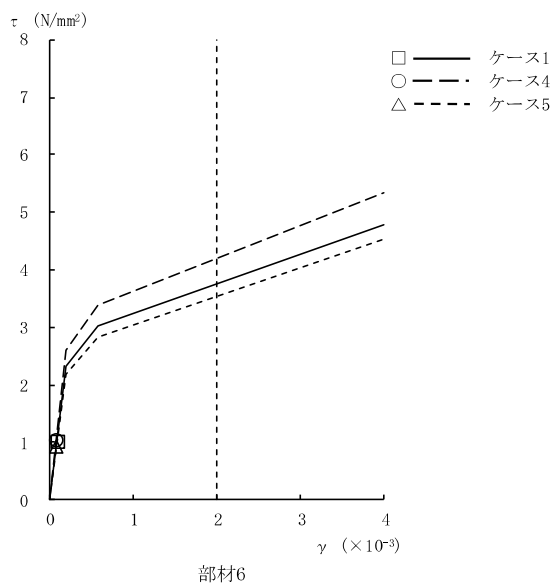
図 2-127 τ - γ 関係と最大応答値 (Ss-3, EW 方向, 1F) (1/4)
