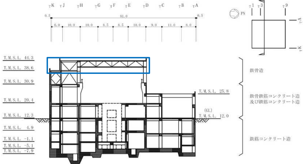
(a) タービン建屋の断面図
