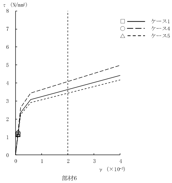
図 2-121 τ - γ 関係と最大応答値 (Ss-1, NS 方向, 1F) (1/4)
