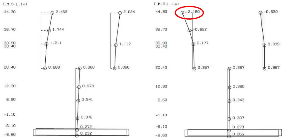
図 2-2(a) 刺激関数図 (ケース 2) (NS 方向, S s -2)
