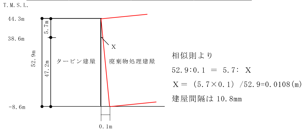
図 5-4 もやの変形を考慮しない場合の建屋間隔
