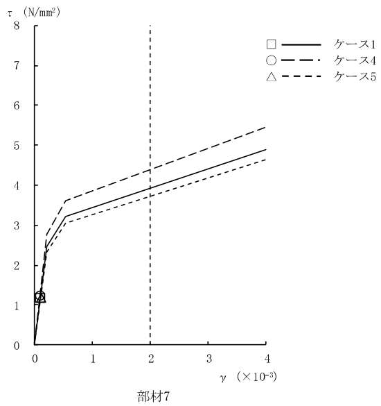
図 2-121 τ - γ 関係と最大応答値 (Ss-1, NS 方向, B1F) (2/4)
