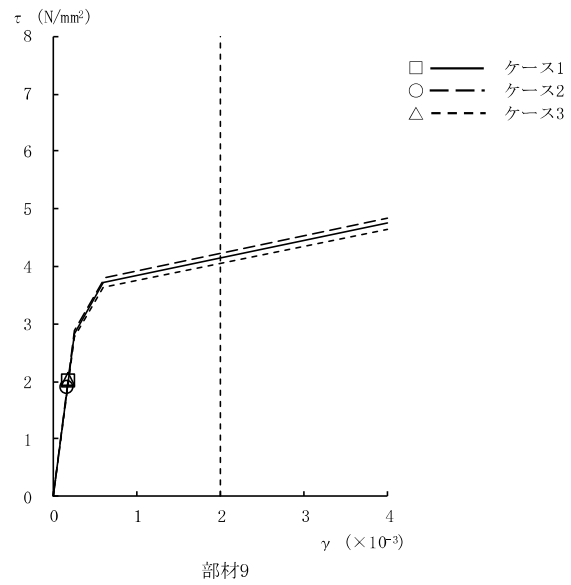
図 2-60 \tau - \gamma 関係と最大応答値 (Ss-8, NS 方向, B3F) (4/4)
