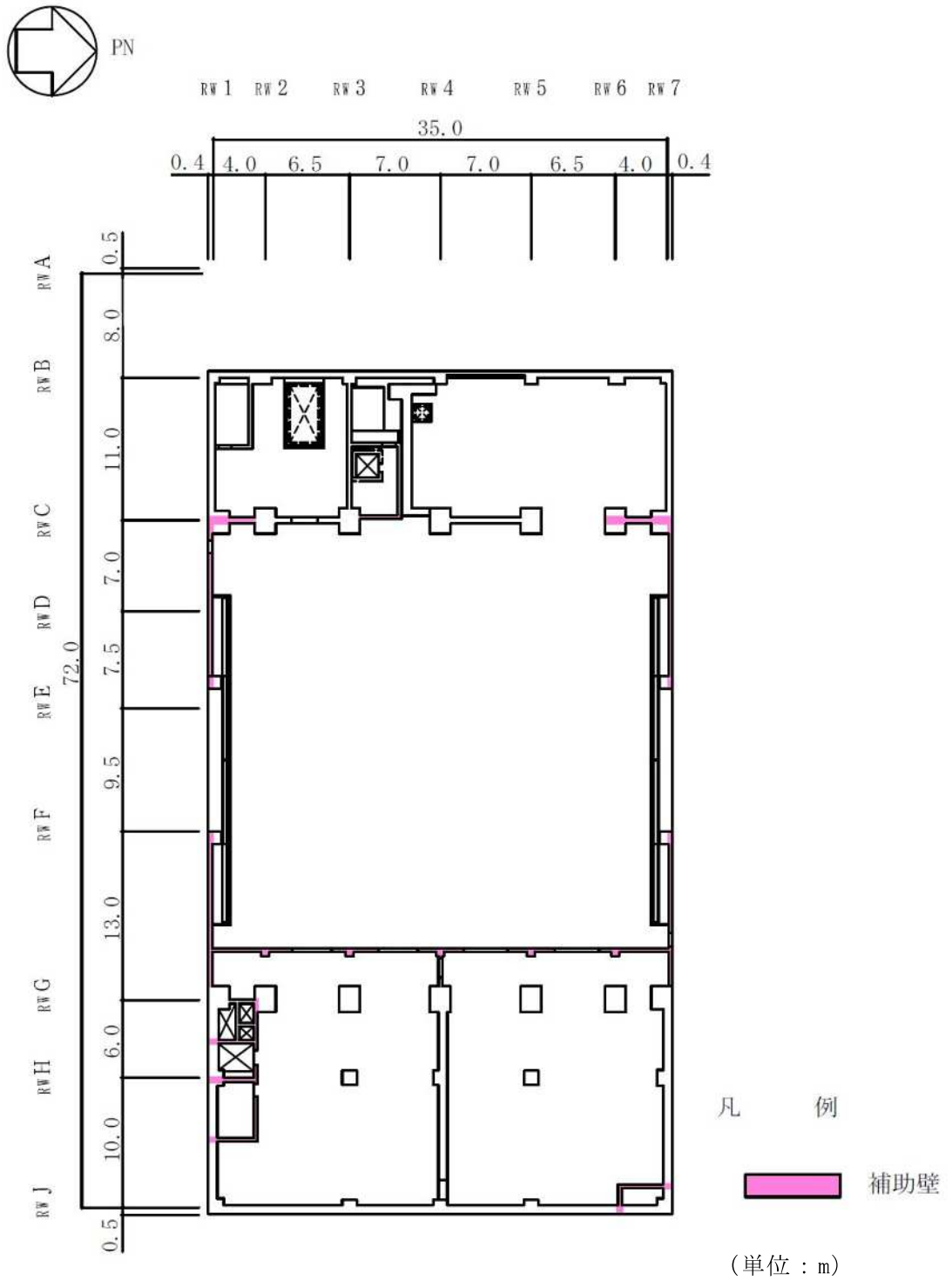
図2-3 補助壁の考慮範囲 (2F, T.M.S.L. 20.4m) (6/6)
