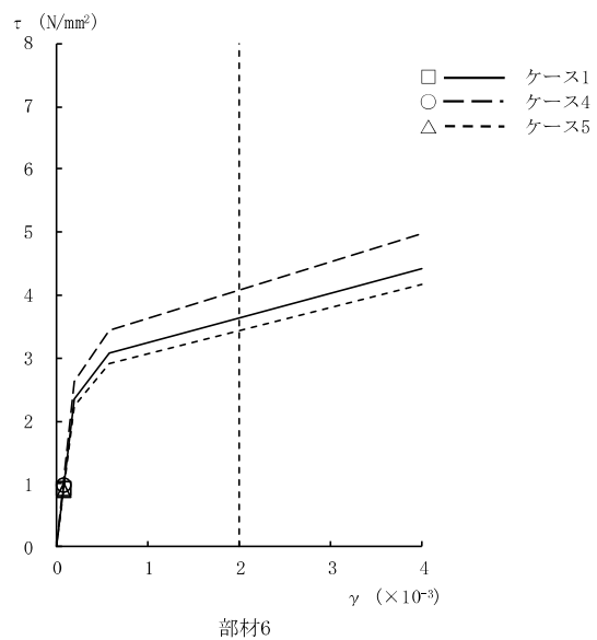
図 2-122 τ - γ 関係と最大応答値 (Ss-2, NS 方向, 1F) (1/4)
