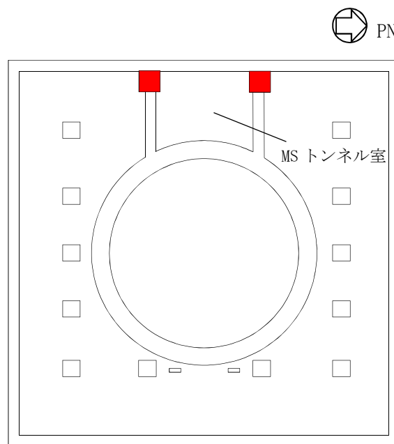
図 1-1 原子炉建屋内側ブローアウトパネル配置図（平面図）
