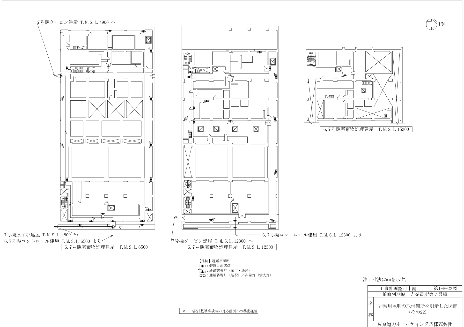
図7 作業用照明の設置場所及び中央制御室から各現場機器室までの移動経路の詳細 13
