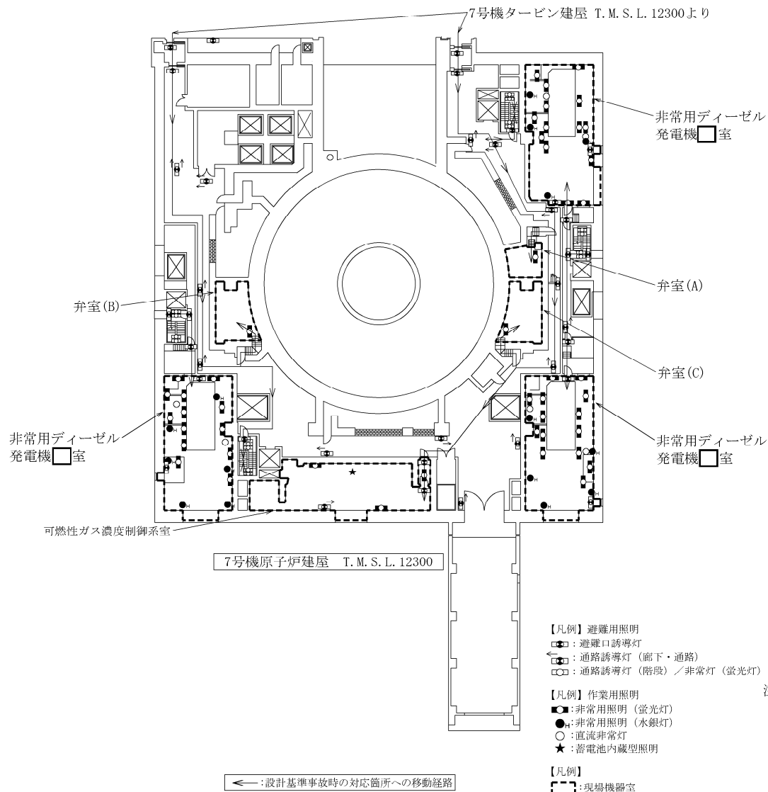
図7 作業用照明の設置場所及び中央制御室から各現場機器室までの移動経路の詳細 4
