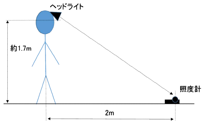
図1 乾電池内蔵型照明（ヘッドライト）の照度確認方法
