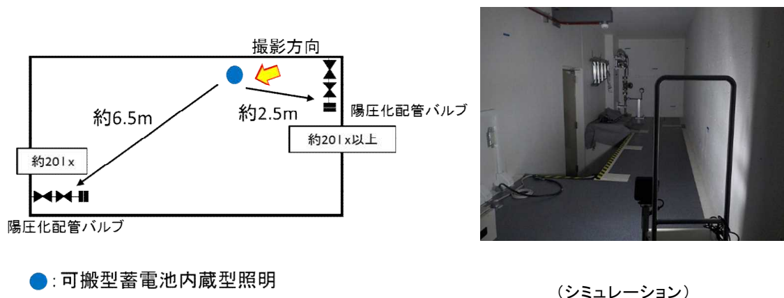
図3 中央制御室待避室における重大事故等発生時の可搬型の照明の照度確認状況
