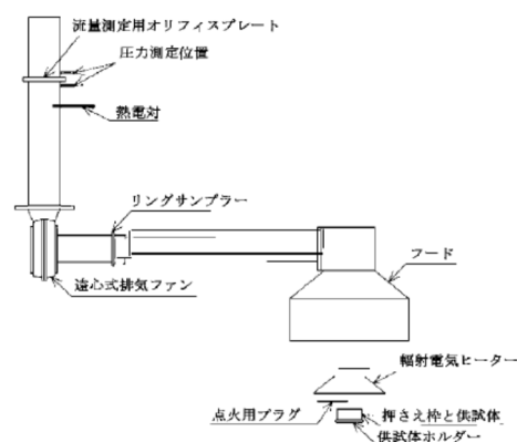
図 3 試験装置の概要
