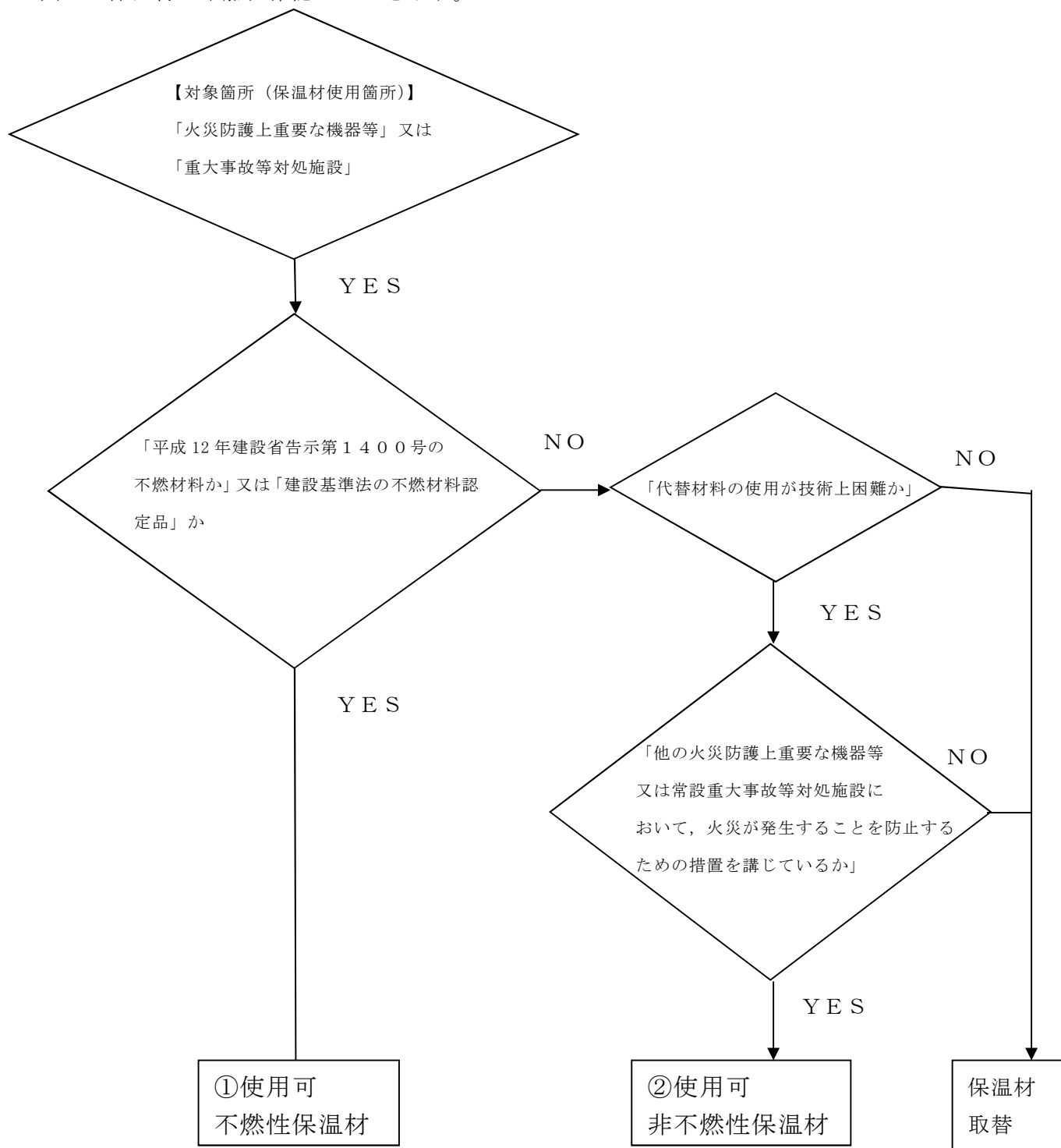
図1 保温材の不燃性確認フロー
