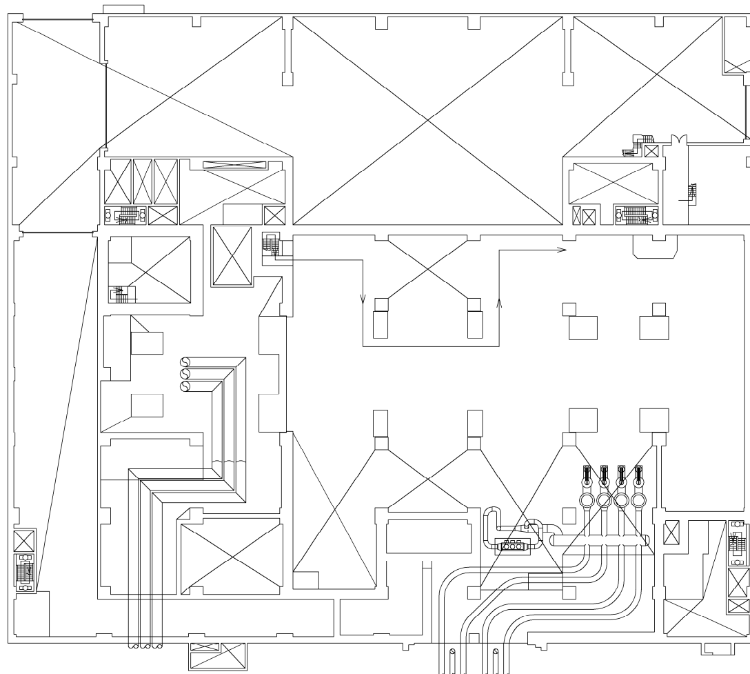
7号機タービン建屋 T.M.S.L. 17000
