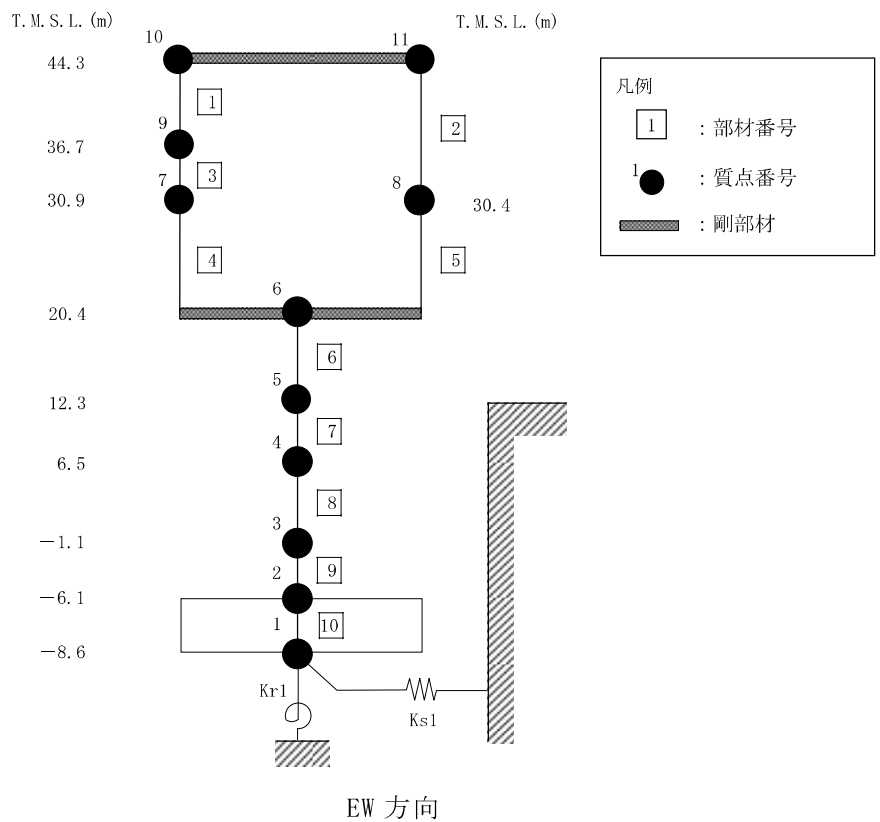
図 4-1 地震応答解析モデル (水平方向) (1/2)
