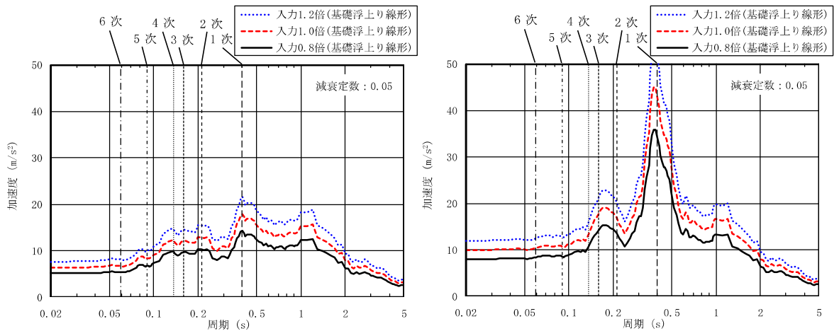
(b) 基礎浮上り線形モデル
