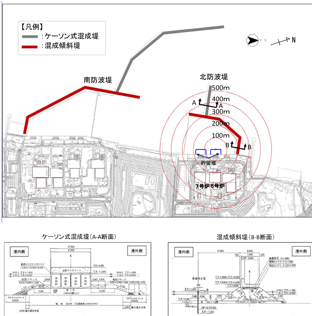
図 4.2-27 防波堤の配置及び構造概要
