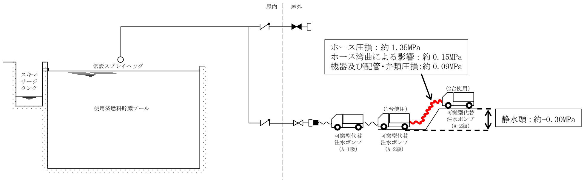
図 4-4 燃料プール代替注水系 使用済燃料貯蔵プールへスプレイする場合（常設スプレイヘッド使用時）
