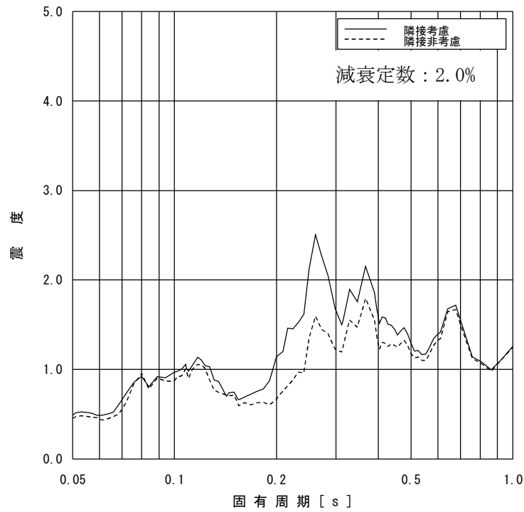
図 2-7 床応答スペクトルの比較 (原子炉遮蔽壁 T. M. S. L. 13. 9500m, 水平方向, 減衰定数 2. 0%)
