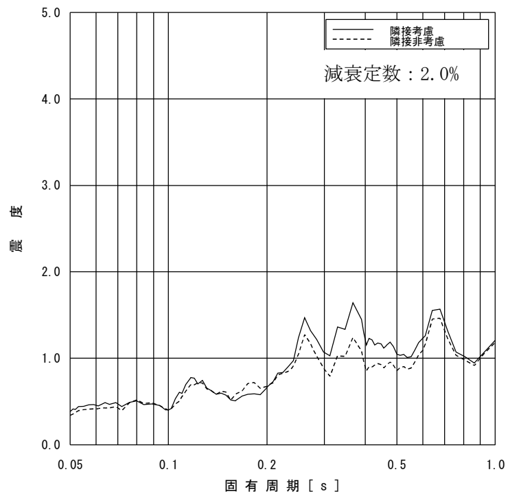
図 2-15 床応答スペクトルの比較 (原子炉本体基礎 T.M.S.L.-4.700m, 水平方向, 減衰定数 2.0%)
