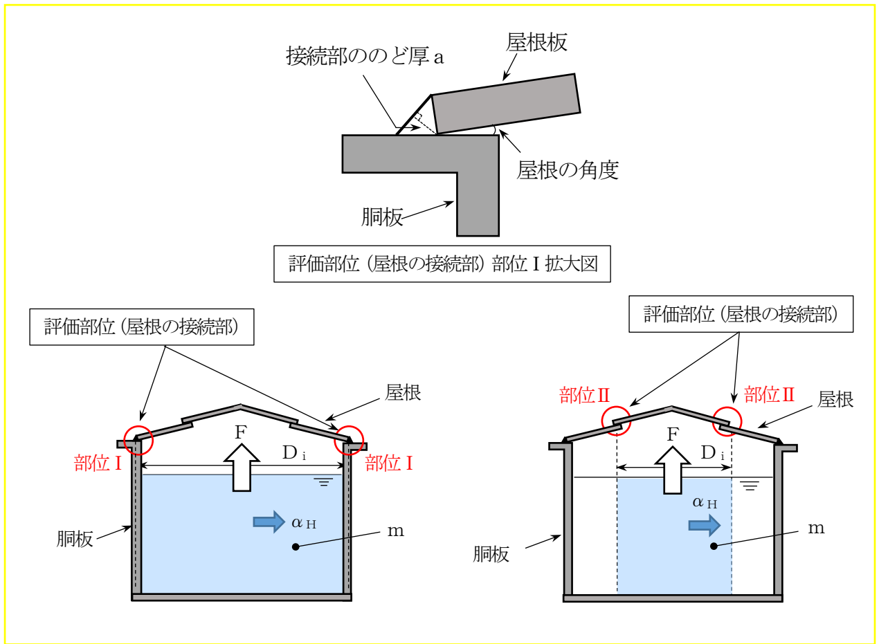
図1 保守的な評価の概略図 (軽油タンクの例)
