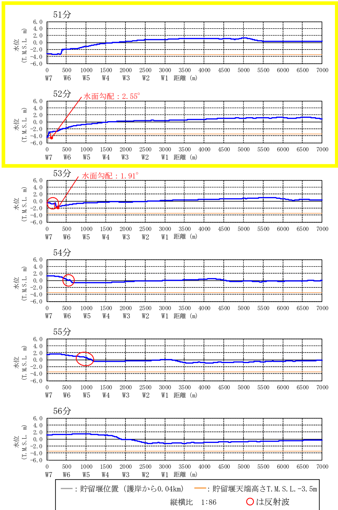
図 4.7 参 1-37 水位の空間分布の時間変化 (基準津波 3) [51-56 分]
