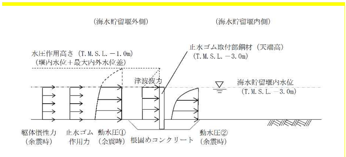
図 2.4-3-9 荷重作用図（止水ゴム取付部鋼材 重畳時 2 北側）
