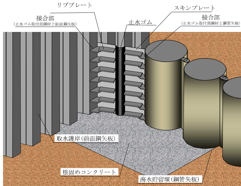
図 2 海水貯留堰接続部（南側）の鳥瞰図
