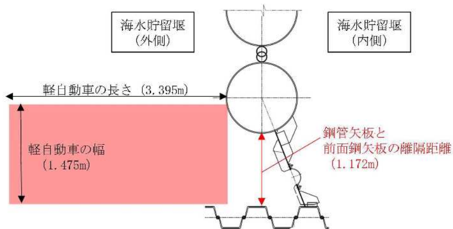
図5 (1) 止水ゴム取付部鋼材に軽自動車近接した時の状況 (平面図)
