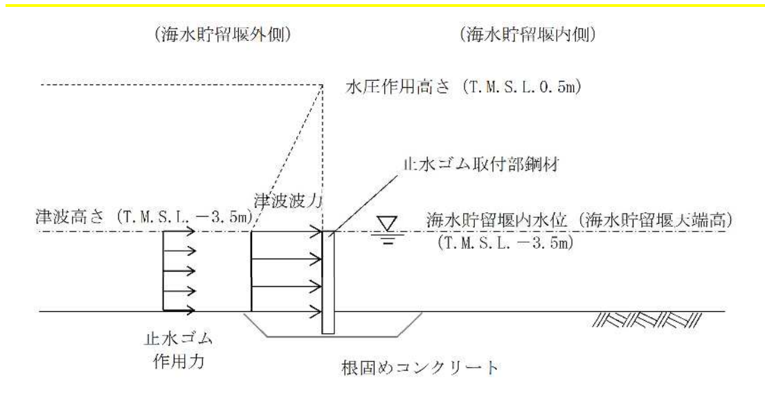
図 2.3-3-6 荷重作用図（止水ゴム取付部鋼材 津波時）
