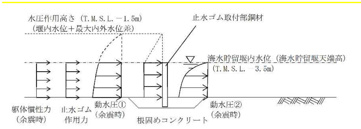
図 2.3-3-8 荷重作用図（止水ゴム取付部鋼材 重畳時 2）
