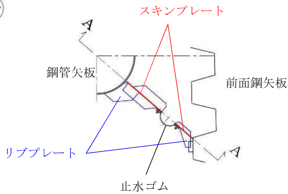
(a) 平面図
