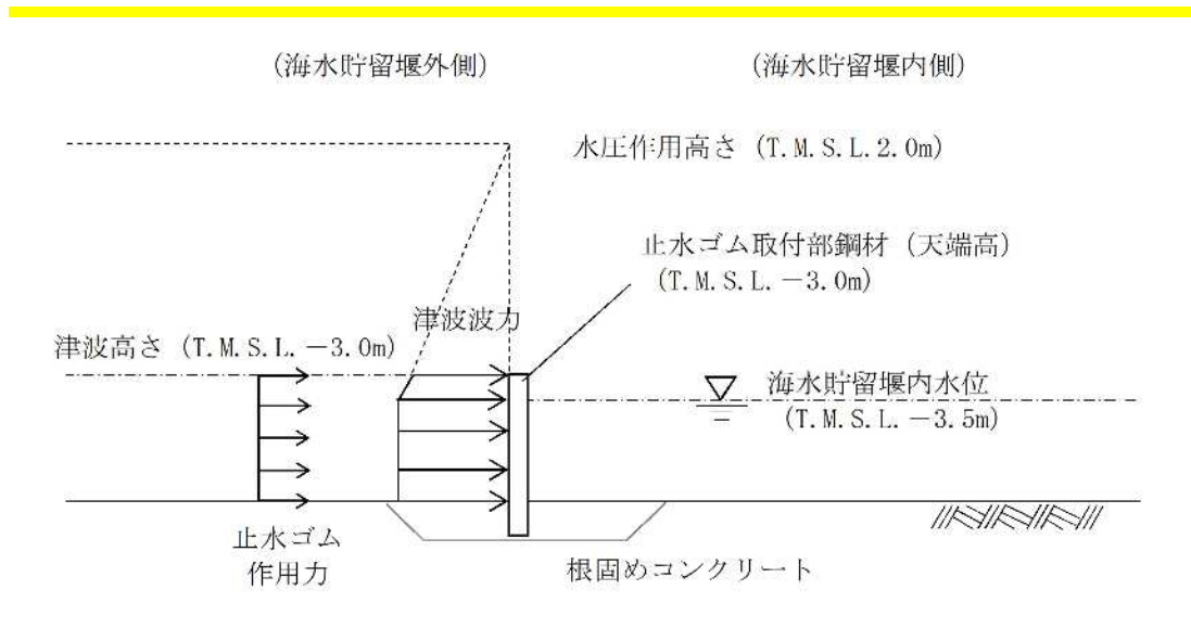
図 2.4-3-7 荷重作用図（止水ゴム取付部鋼材 津波時 北側）
