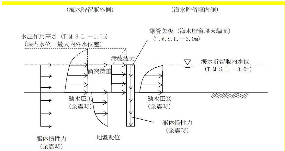
図 2.4-3-6 荷重作用図（鋼管矢板 重畳時 2 北側）
