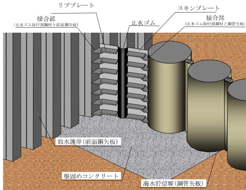
図 2.3-3-12 海水貯留堰接続部の鳥瞰図
