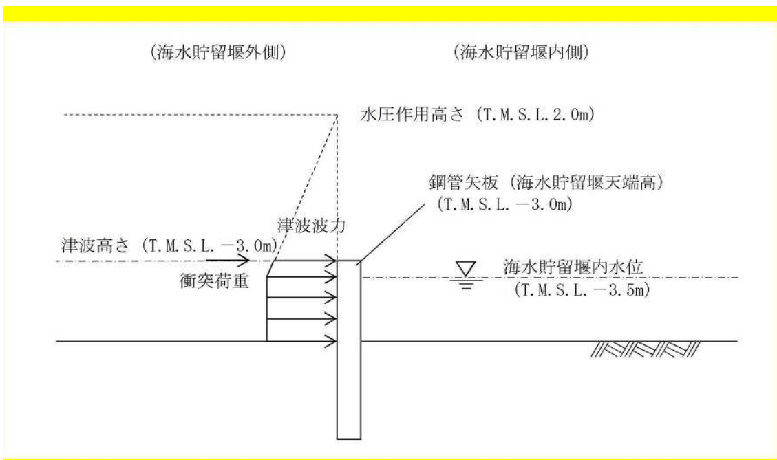
2.4-3-4 荷重作用図 (鋼管矢板 津波時 北側)
