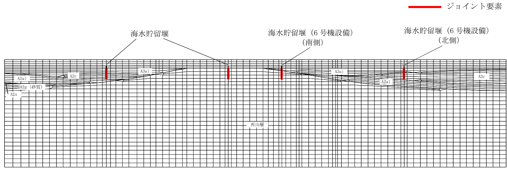
図 2.2-3-18 (2) ジョイント要素の配置 (B-B断面)
