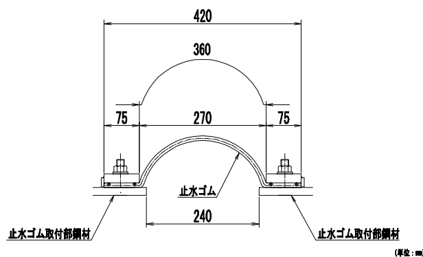
図 15 止水ゴム構造図
