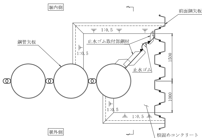
図1 根固めコンクリートの形状（平面図）
