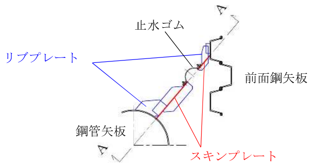
(a) 平面図
