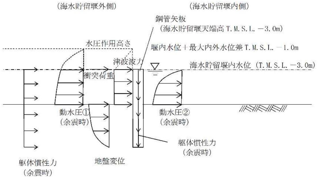
図 3-6 荷重作用図 (鋼管矢板 重畳時 2 北側)
