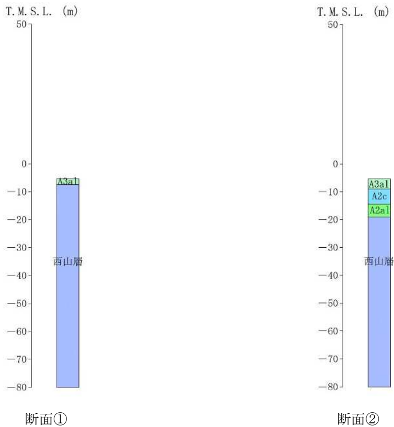
図 3-3(2) 評価対象断面図
