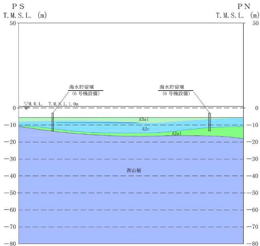
图 3-2(2) 地質断面図 (B-B断面図)
