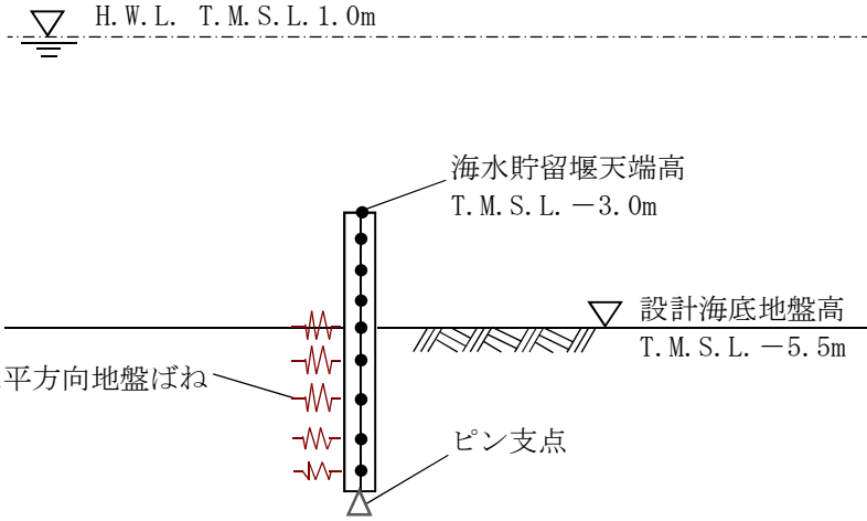
図 3-10 解析モデル
