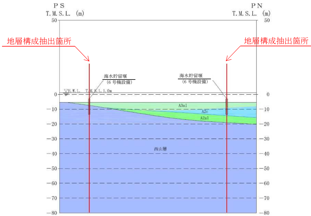
図 3-3(1) 地質断面図 (A-A断面図)
