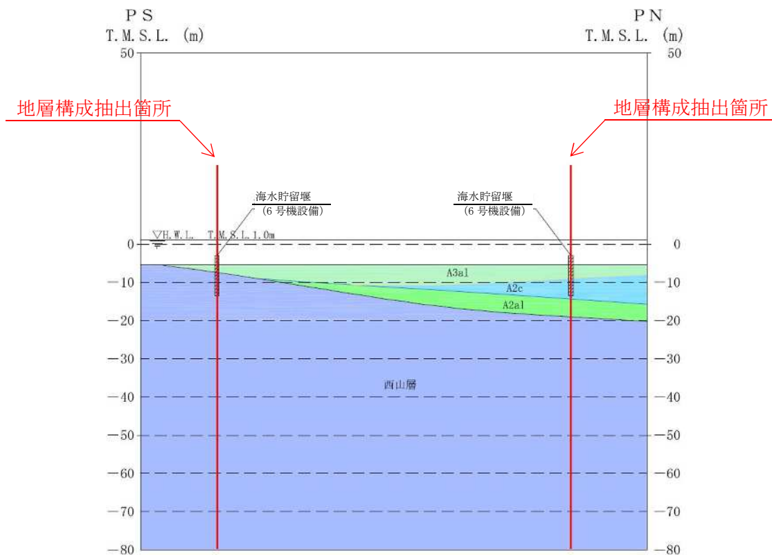
图 3-2(1) 地質断面図 (A-A断面図)
