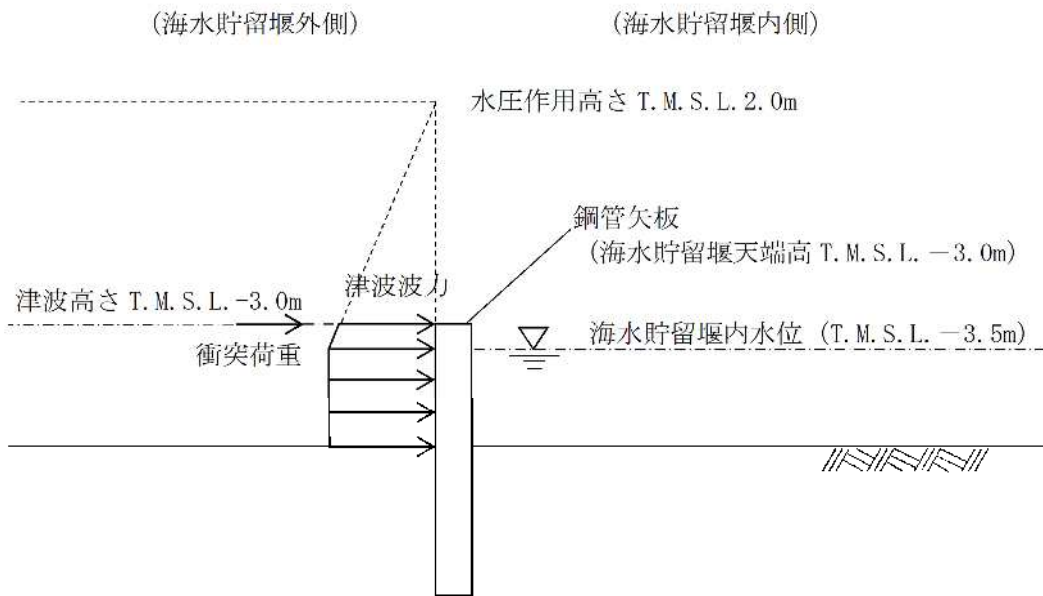
図 3-4 荷重作用図 (鋼管矢板 津波時 北側)
