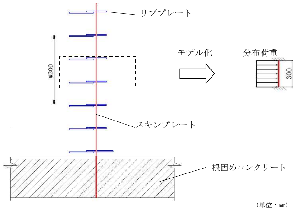
図 3-12 照査モデル図（スキンプレート）
