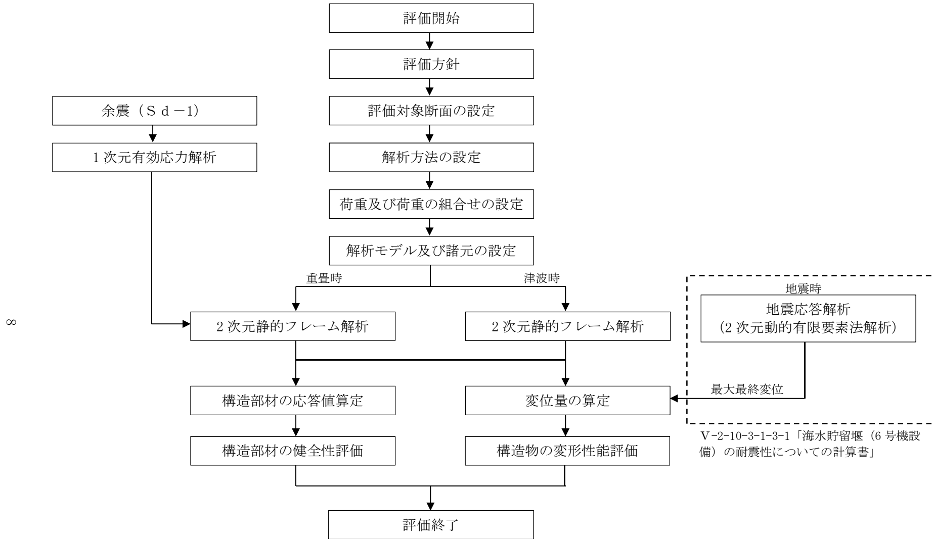
図 2-4 海水貯留堰（6号機設備）の強度評価フロー
