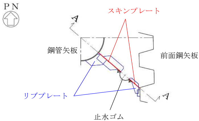
(a) 平面図
