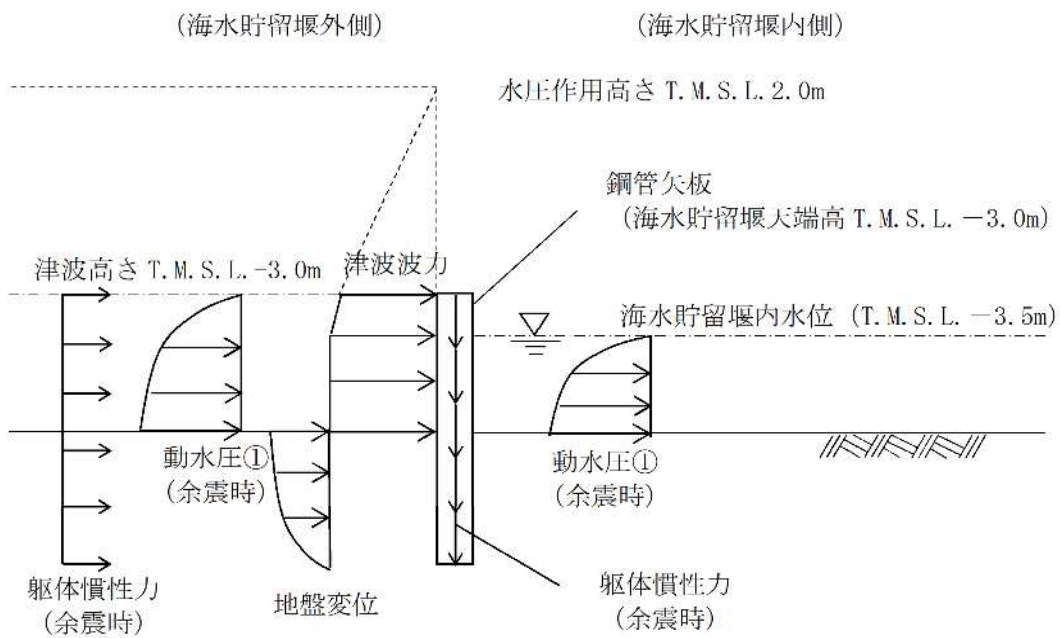
図 3-5 荷重作用図 (鋼管矢板 重疊時 1 北側)
