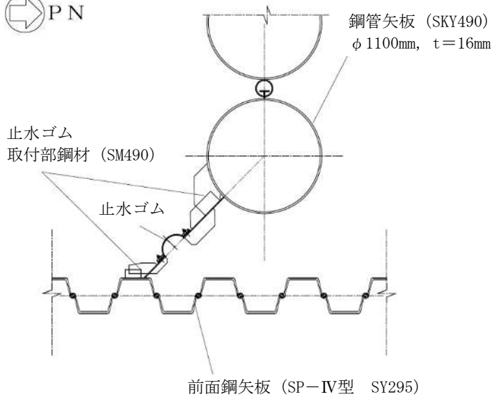
図 2-2(2) 海水貯留堰 (6号機設備) の平面図 (A部拡大)
