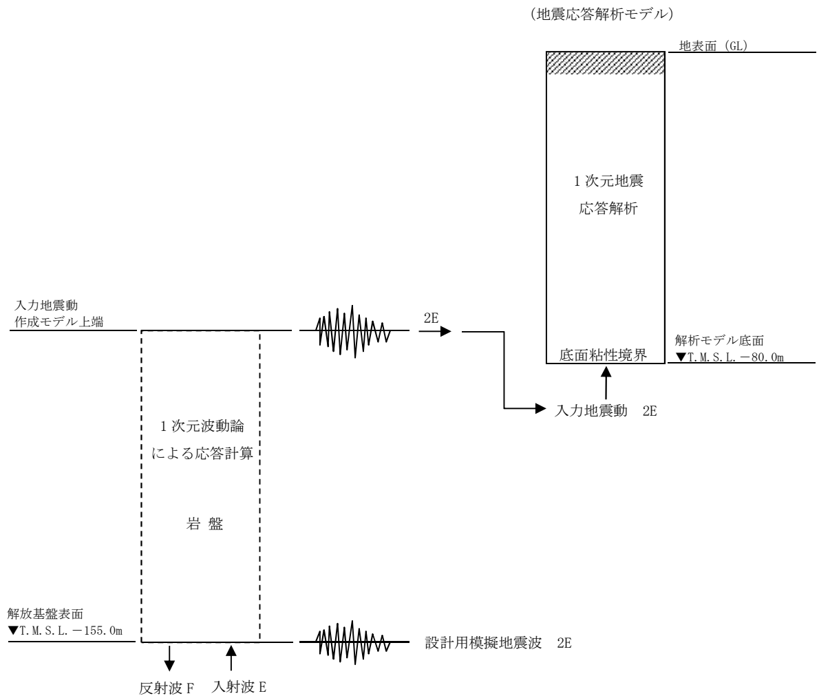
図 3-20 入力地震動算定の概念図
