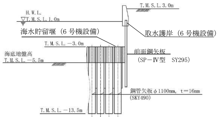
(a) A-A 断面図
