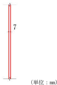
図 3-12 照査モデル図（スキンプレート）
