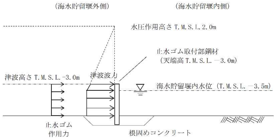
図 3-7 荷重作用図 (止水ゴム取付部鋼材 津波時 北側)
