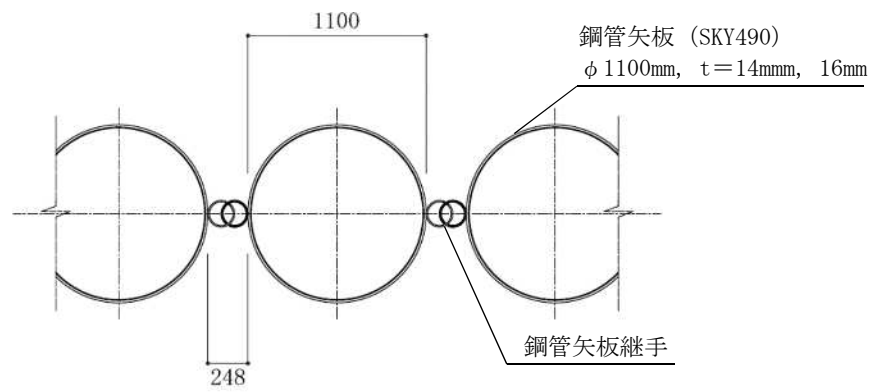
a. P-P 継手
