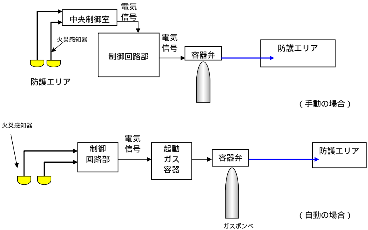
図 5 - 8 小空間固定式消火設備（選択弁なし）、SLC ポンプ・CRD ポンプ局所消火設備、5号機原子炉建屋内緊急時対策所消火設備 系統構成
